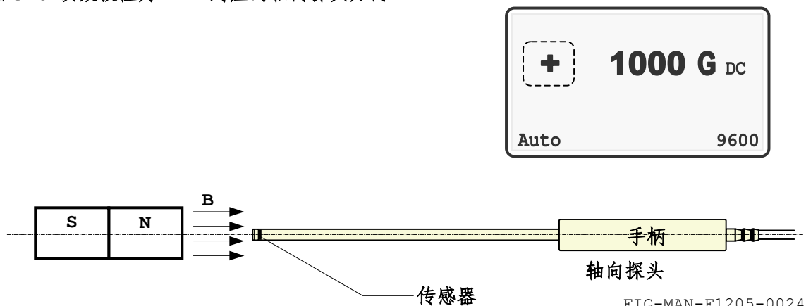
图 3-6 读数极性为“+”对应的轴向探头方向
