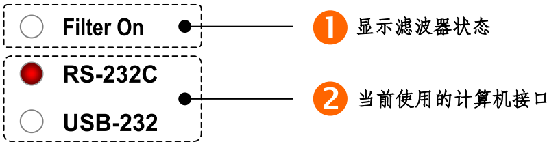
图 3-3 F1205 的 LED 指示器
