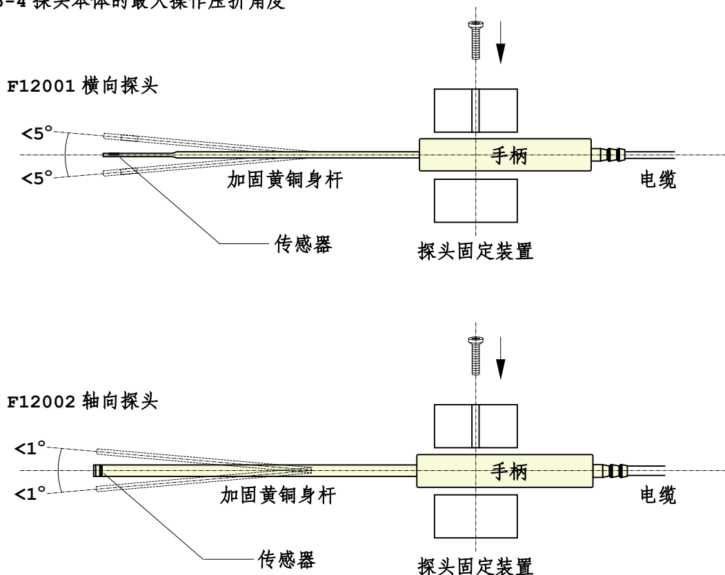
图 5-4 探头本体的最大操作压折角度
