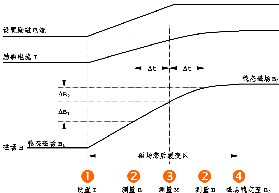
图 3-14 滞后现象造成的测量时差 \Delta t
