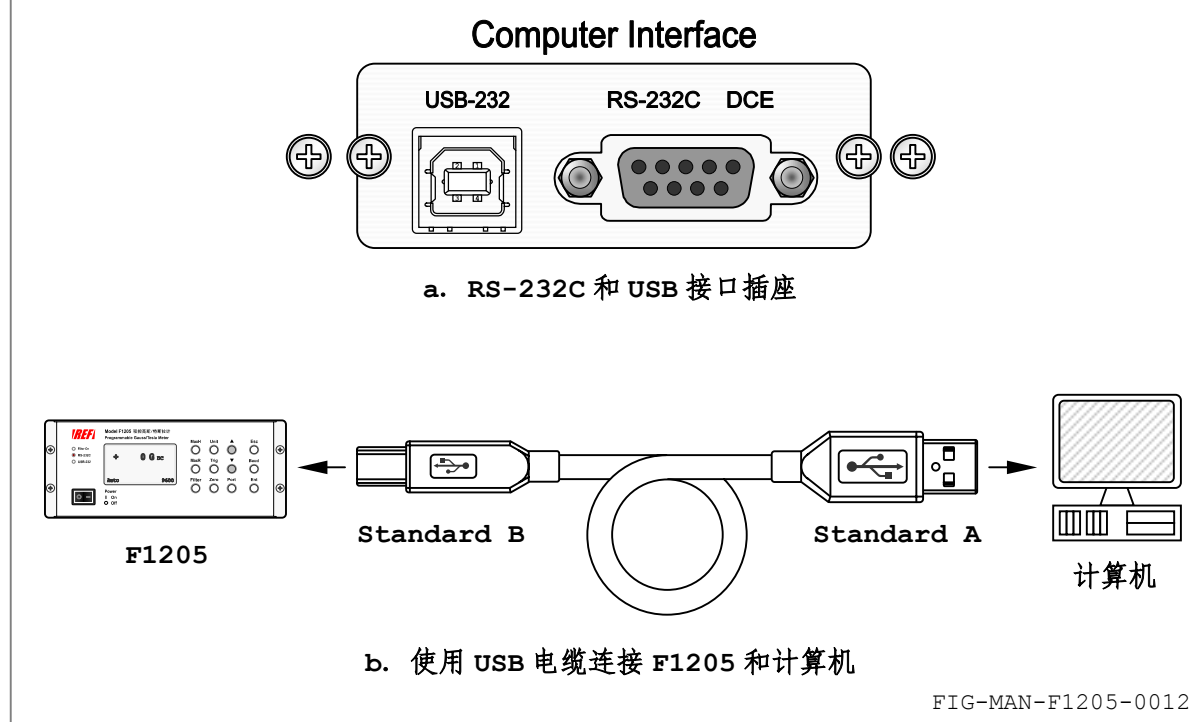
图 2-8 计算机接口连接器以及使用 USB 电缆连接 F1205 和计算机
