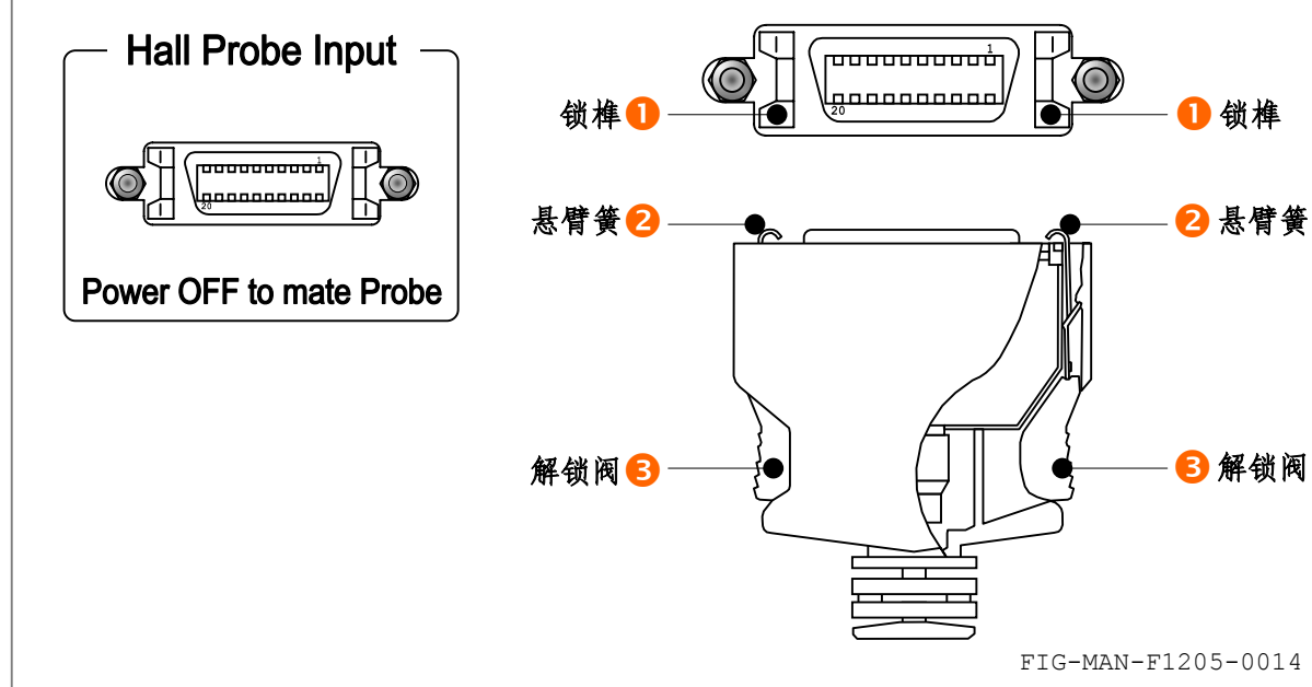
图 2-9 探头接口和探头连接方法
