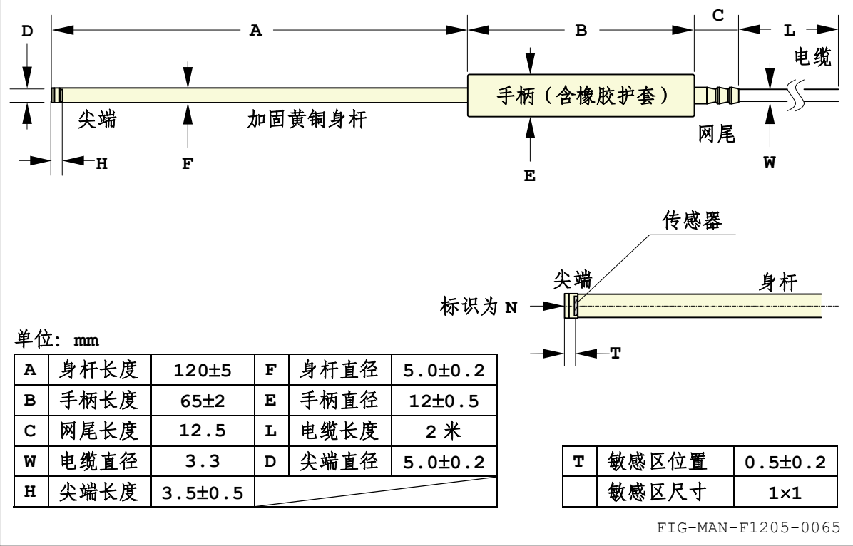
图 5-2 F12002 通用数字化轴向霍尔探头二视图
