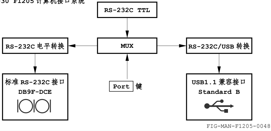
图 3-30 F1205 计算机接口系统
