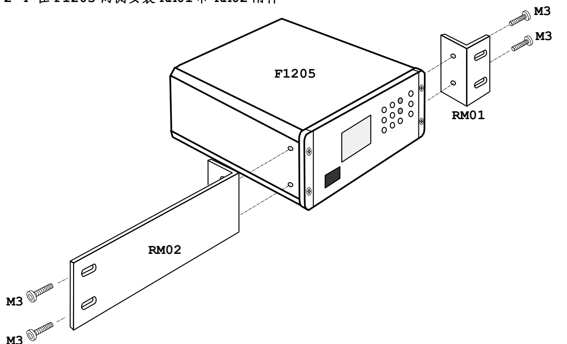
图 2-4 在 F1205 两侧安装 RM01 和 RM02 附件
