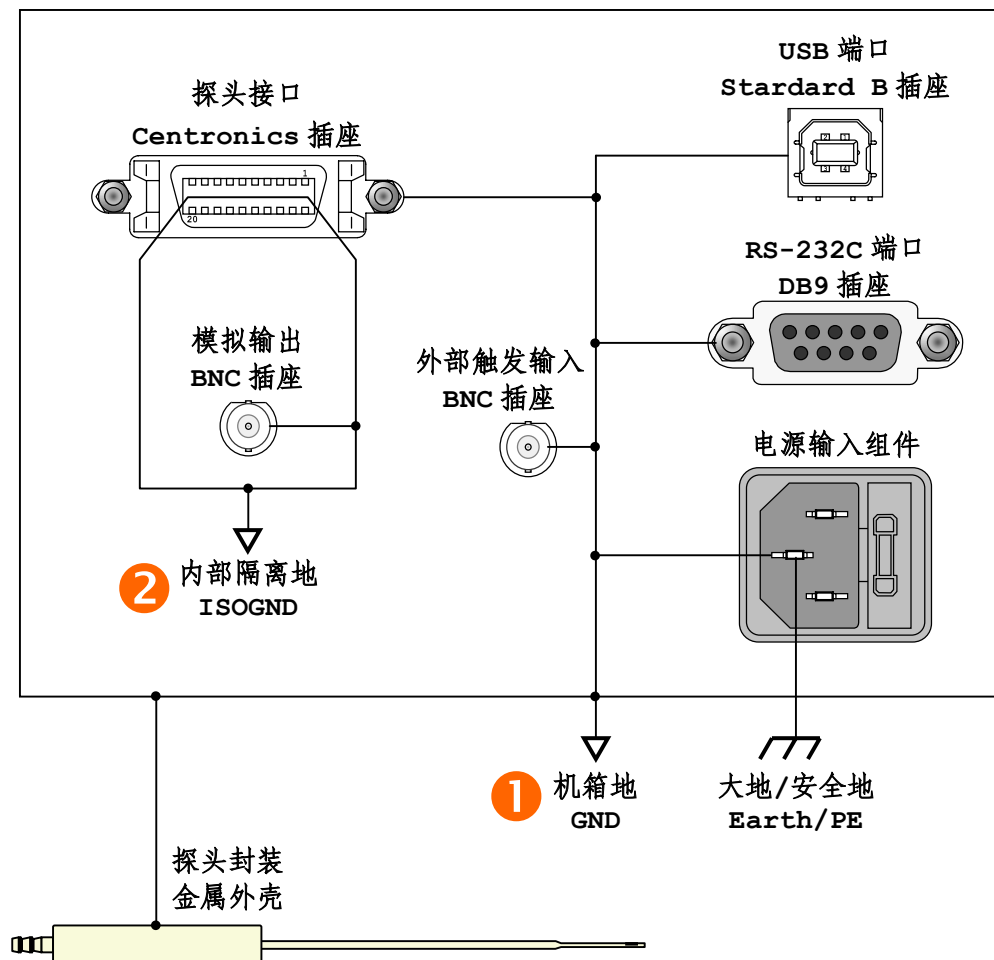
图 3-41 F1205 的接地关系
