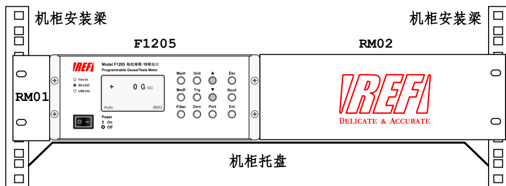
图 2-5 F1205 与机柜的连接安装方法
