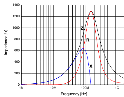
SHB-1M1608-102J HB-1M1608-102J
