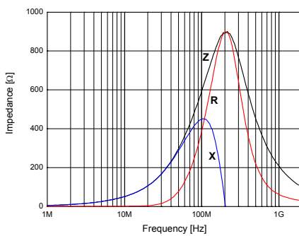
SHB-1M1608-601J
