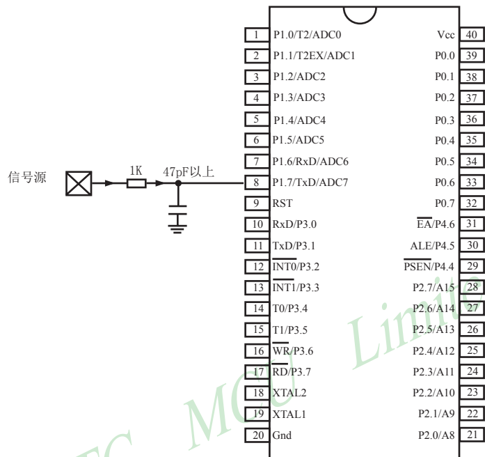
A/D转换在P1口, P1.0 - P1.7共8路
