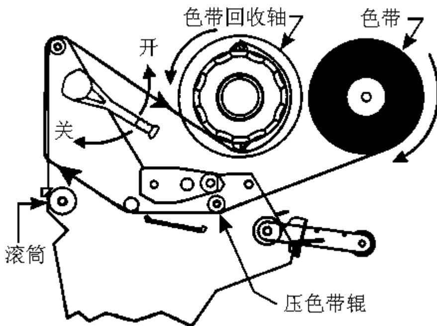
[色带安装图]
