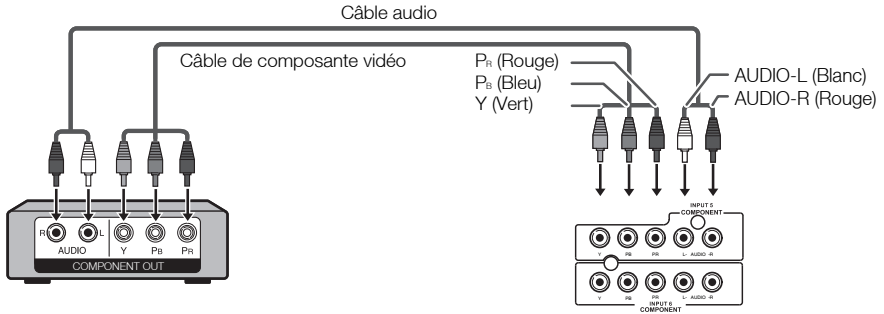
Panneau arrière Entrées horizontales
