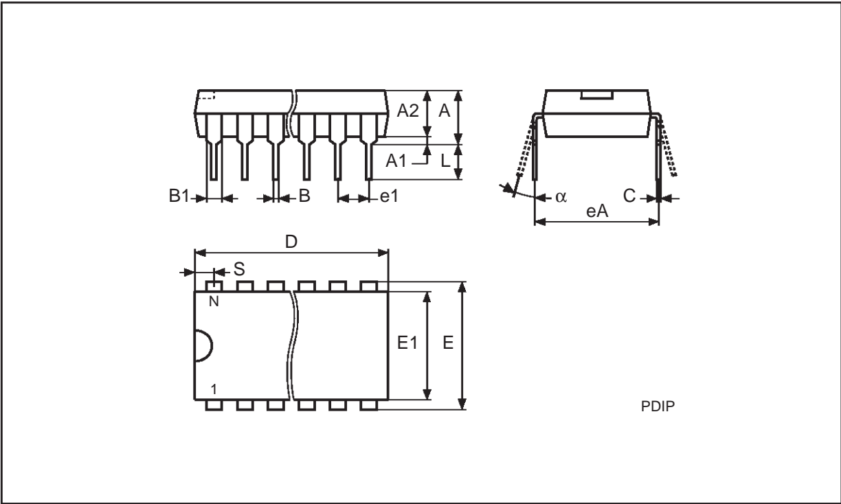
PDIP24
