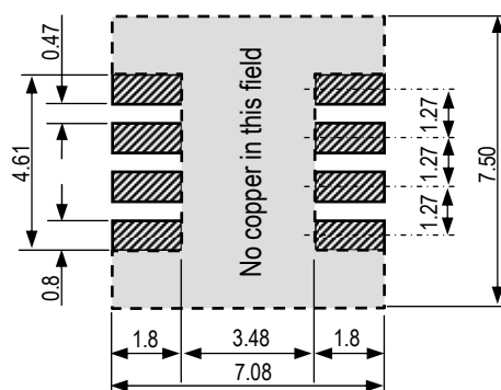
图 7: 推荐 SHT1x 引脚尺寸, 单位 mm.
