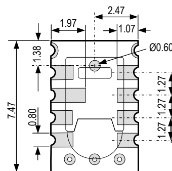
图 6: 传感器电极的后面, 俯视图.
