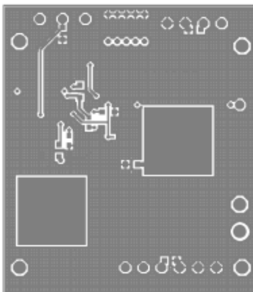
BOTTOM LAYER
