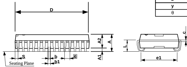
SOJ - 28
