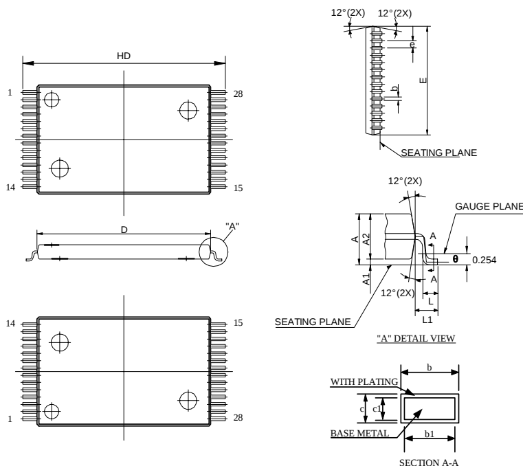
TSOP - 28
