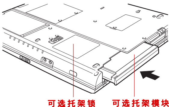
图 4-5 装入辅助硬盘盒示意图
