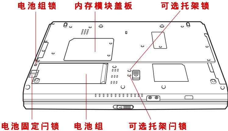
图 2-5 电脑的底部面板部件示意图
