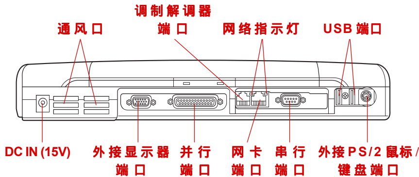
图 2-4 电脑的后侧面板部件示意图
