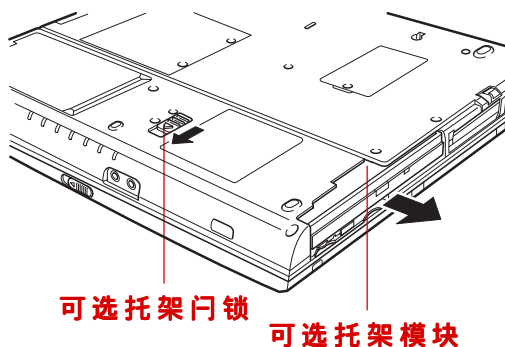
图 4-4 移除 DVD-ROM 驱动器示意图
