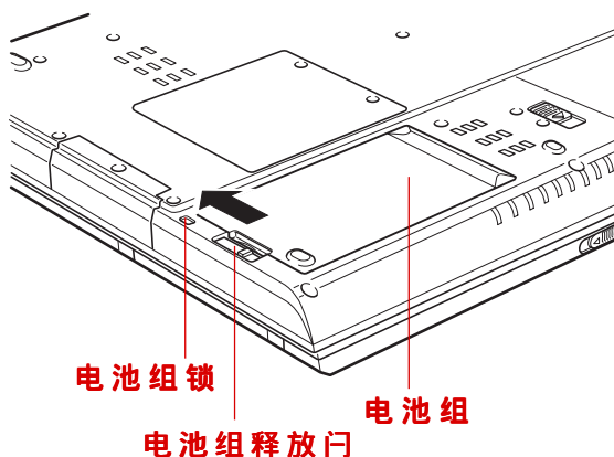
图 6-1 移除电池组示意图
