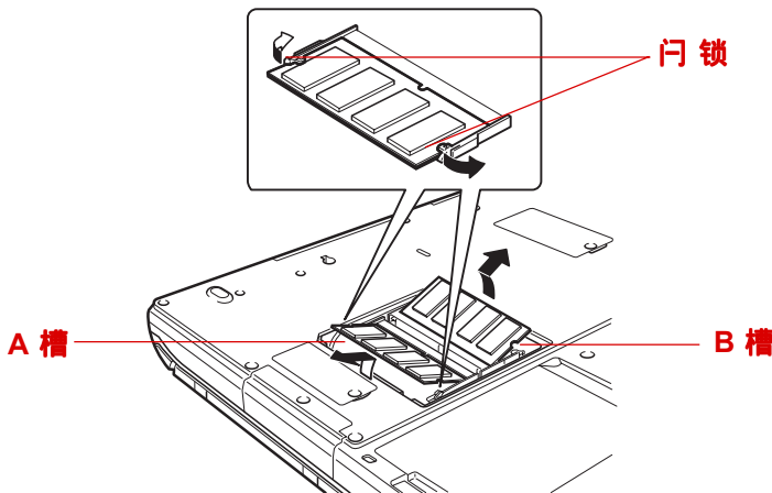
图 8-6 移除内存模块示意图
