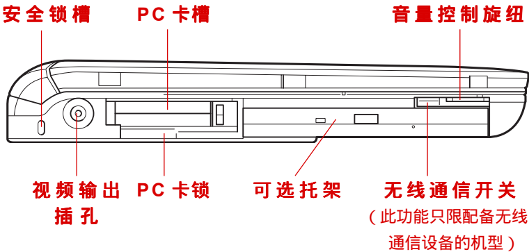
图 2-2 电脑的左侧面板部件示意图
