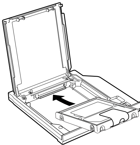
图 8-8 将辅助硬盘装入硬盘盒示意图
