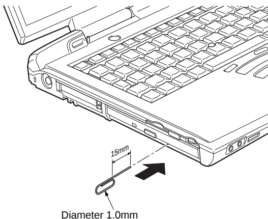
图 4-7 通过退出孔手工打开托盘示意图
