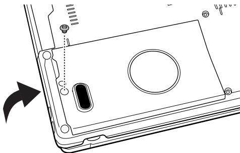
图 8-15 取下硬盘盖板
