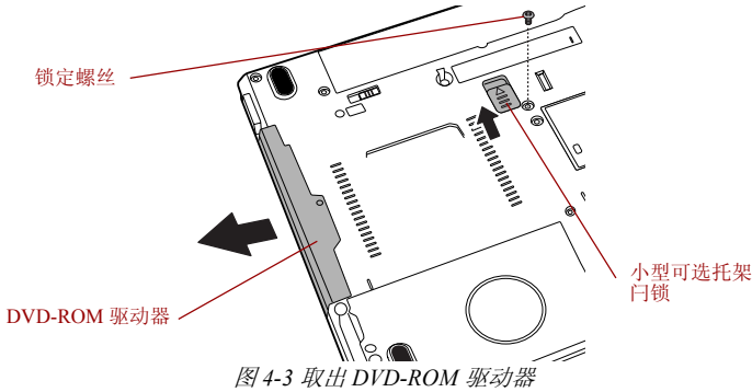
图 4-3 取出 DVD-ROM 驱动器
