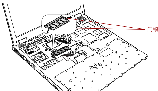
图 8-10 取出内存模块
