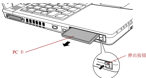
图 8-2 取出 PC 卡
