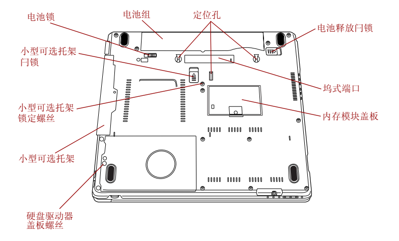
图 2-5 电脑的底部
