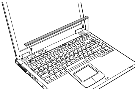
图 8-6 撬开键盘支架，拧出两颗螺丝
