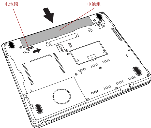
图 6-2 固定电池组
