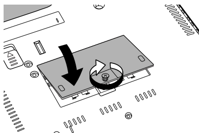
图 8-13 合上内存模块插槽盖
