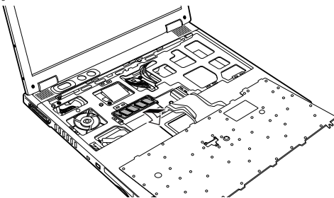
图 8-9 安装内存模块
