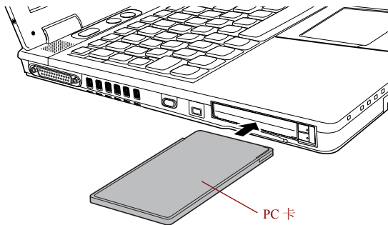
图 8-1 插入 PC 卡
