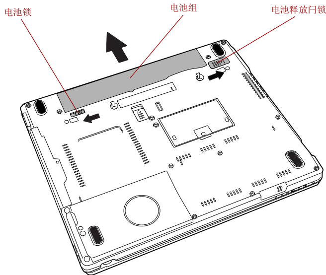
图 6-1 释放电池组
