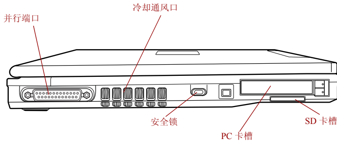
图 2-2 电脑的左侧
