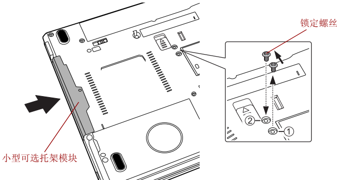
图 4-4 插入小型可选托架硬盘适配器
