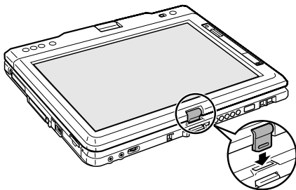
图 4-10 切换到输入板模式(4)
