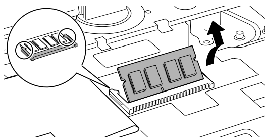
图8-14 取下内存模块
