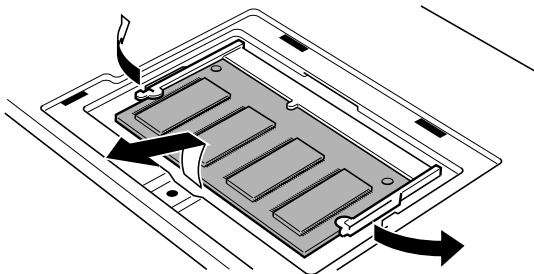
图8-21 取出内存模块
