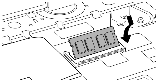
图8-15 安装内存模块于A槽(1)
