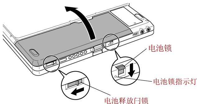
图6-1 取出电池组 (1)
