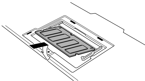
图 8-18 安装内存模块（1）
