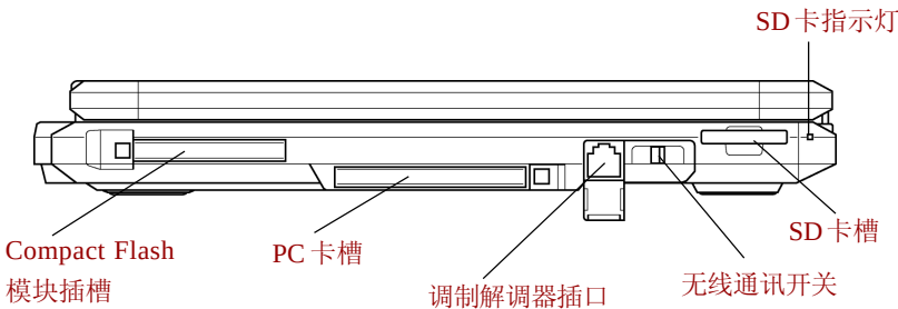
图 2-2 电脑的左侧
