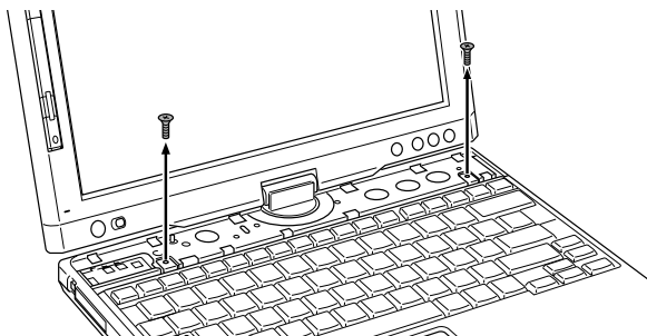
图 8-10 取下键盘支架（1）
