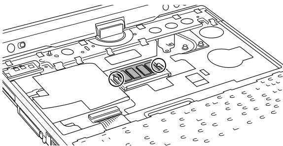
图8-16 安装内存模块于A槽(2)
