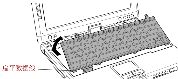
图8-11 取下键盘（2）
