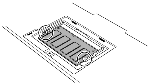
图 8-19 安装内存模块 (2)
