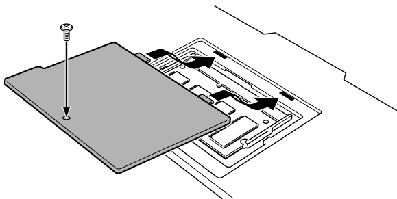
图 8-20 安装内存模块 (3)
