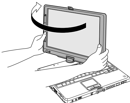
图 4-8 切换到输入板模式(2)
