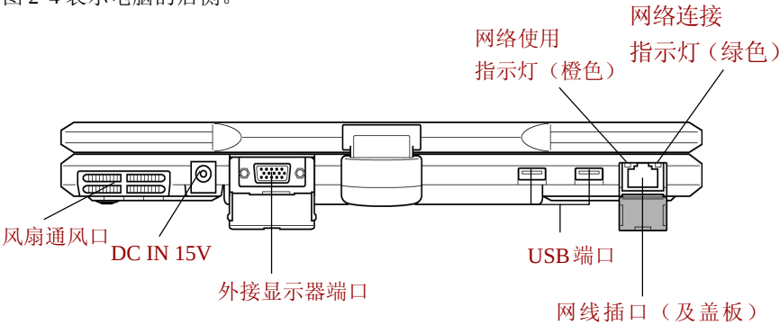
图2-4 电脑的后侧
