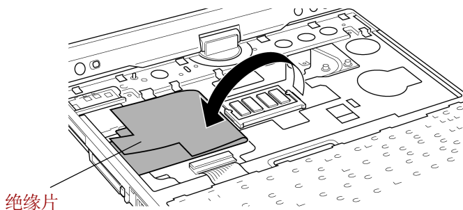
图8-13 揭开绝缘片
