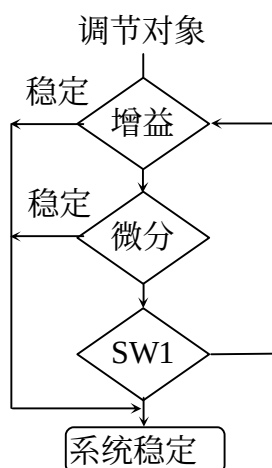
图四.稳定性调整流程
