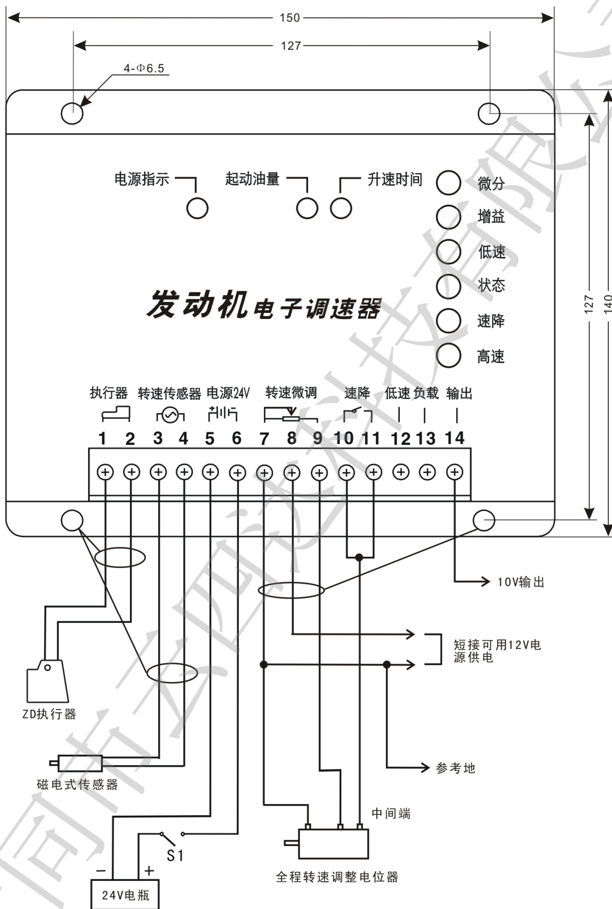
图三.628 系列控制器用于发电机全程调速接线图
