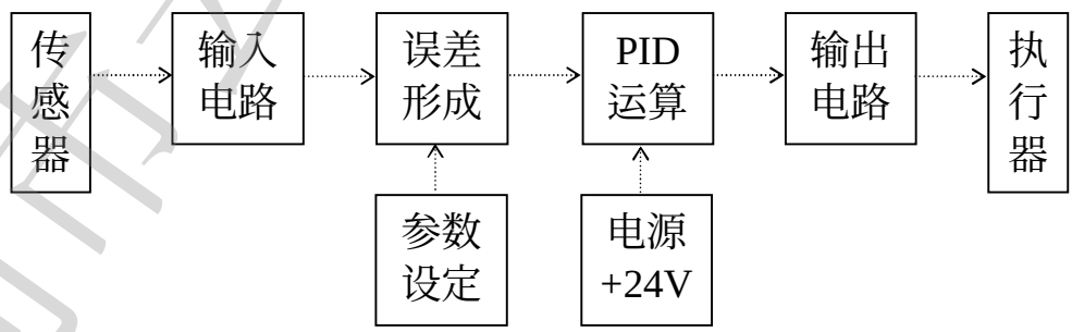
图一. 控制器组成
