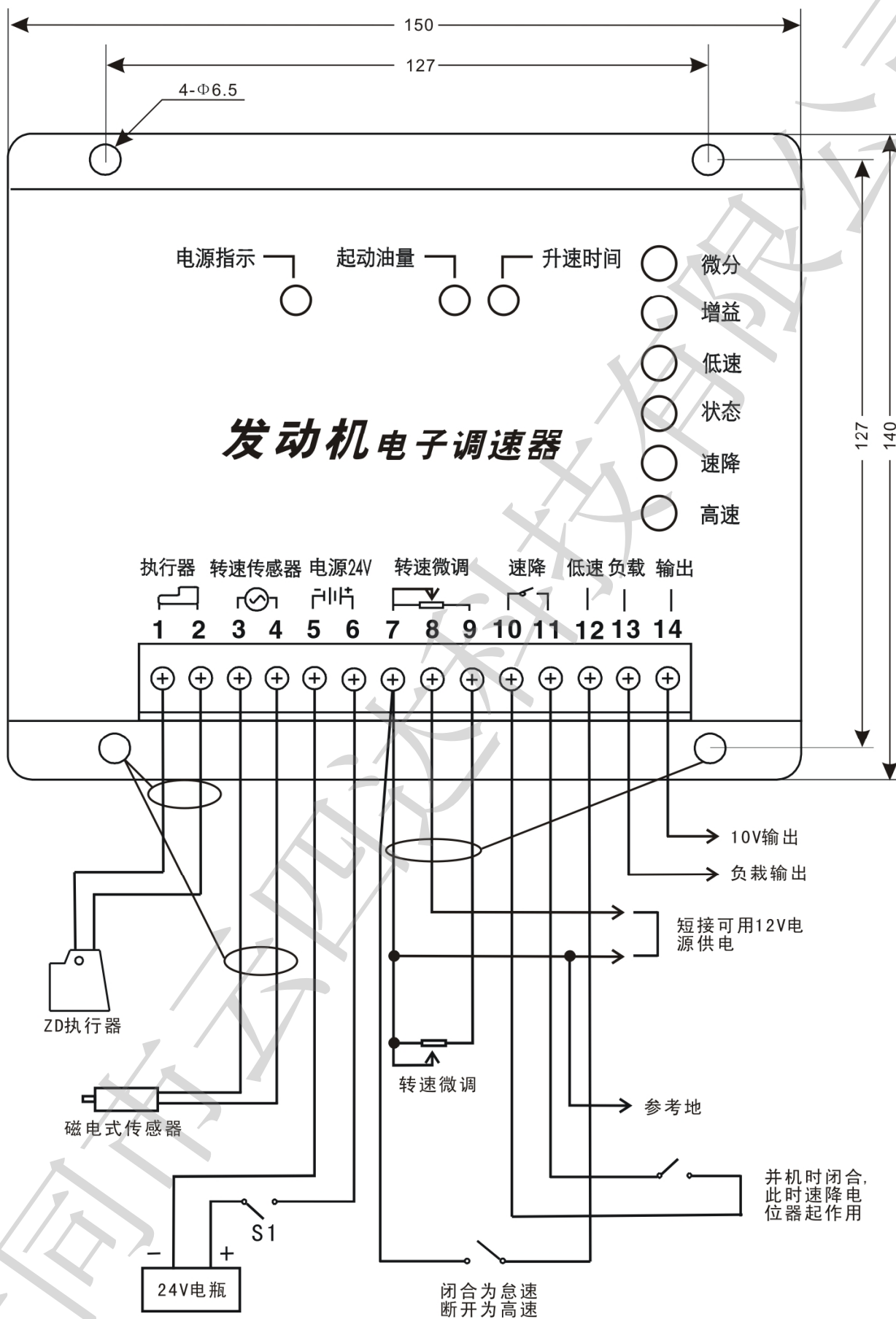
图二.628 系列控制器用于发电机组安装接线图
