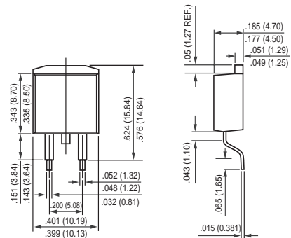
D2PAK
