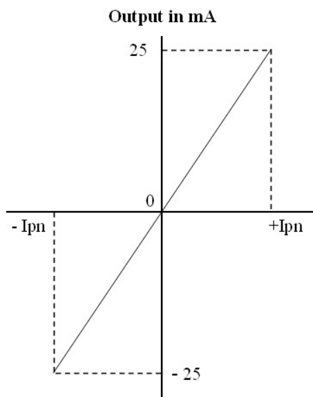
(图 1: 0±25mA 输出)
