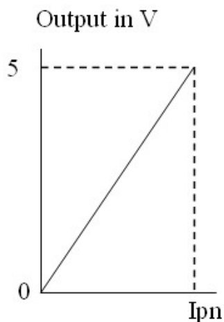
(图 2: 0-5VDC 输出)
