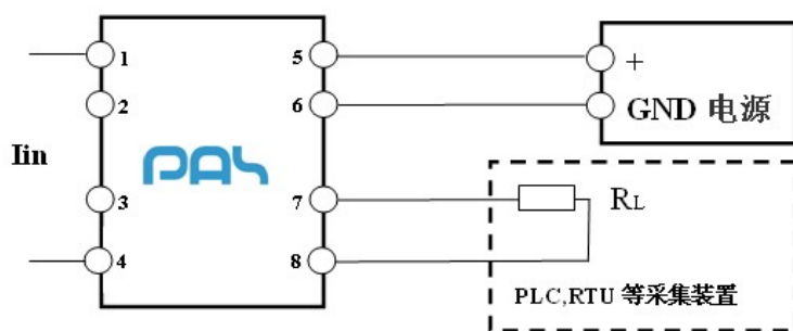
接线示意图
