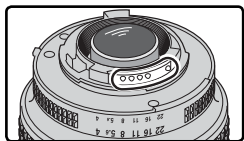
CPU 镜头带有 CPU 接口端子
