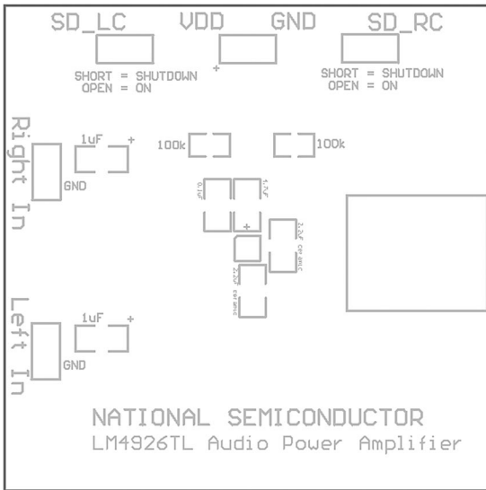
Top Overlay
