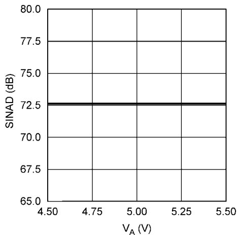
SINAD vs. V_A
