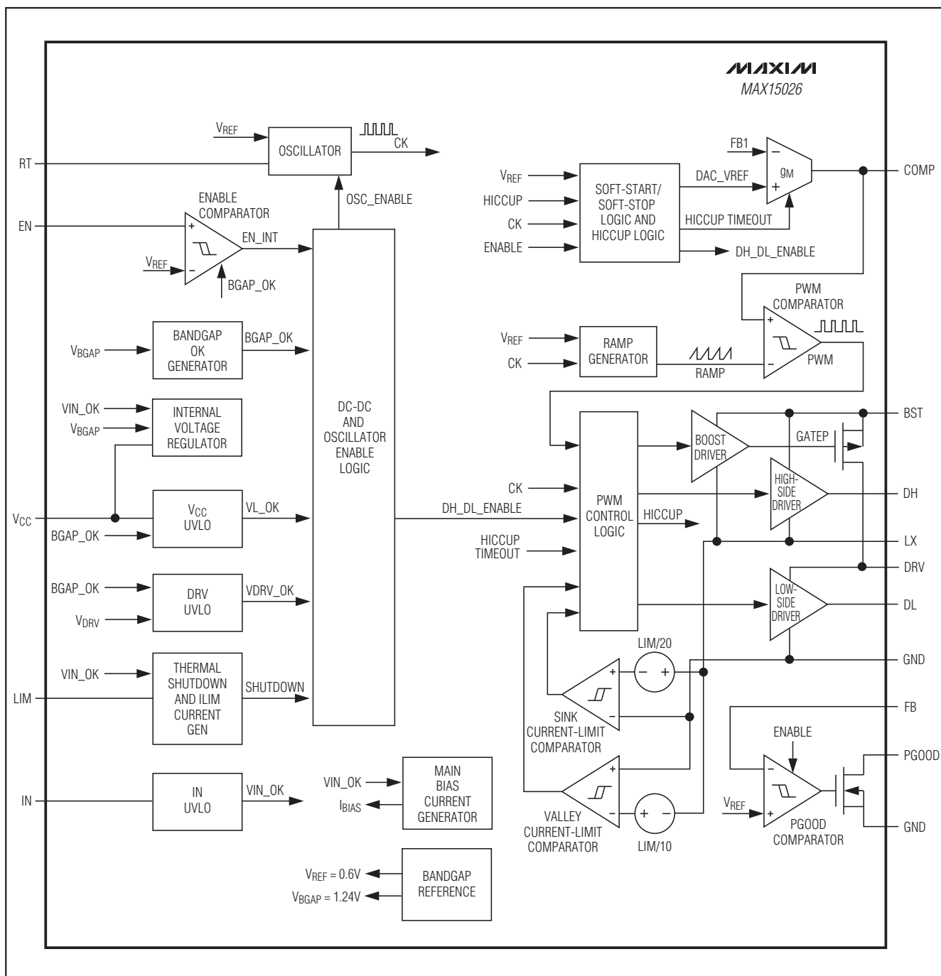
功能框图
