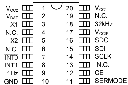
TSSOP (4.4mm)
