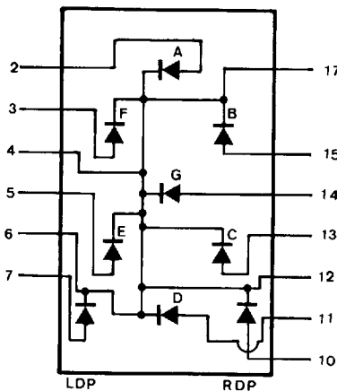
B. LTS-3403L x
