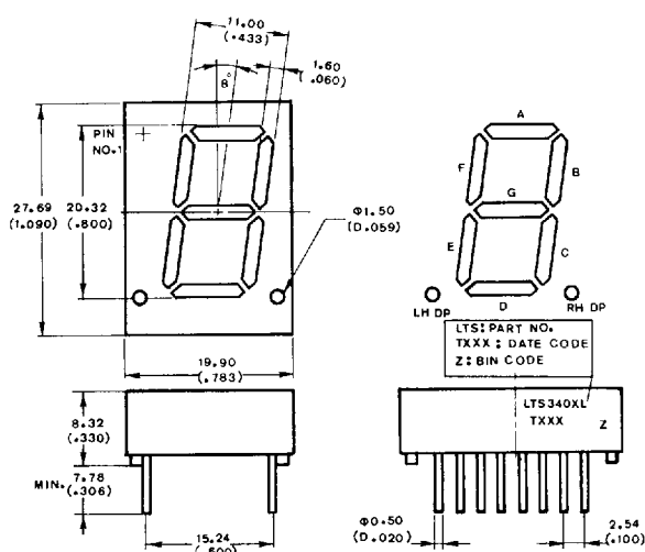
A. LTS-3401 L/3403L
