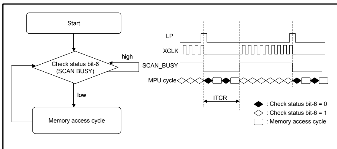
图 6-74 : 以 Check BUSY 来消除雪花的理想状况 (1)
