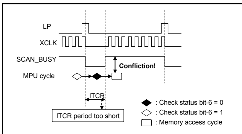
图 6-78 : ITCR 周期过短造成以 Check BUSY 来消除雪花效果不理想 (2)
