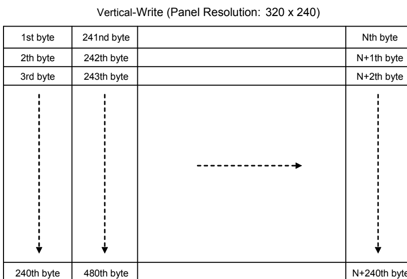
图 6-47 : 垂直数据写入的顺序
