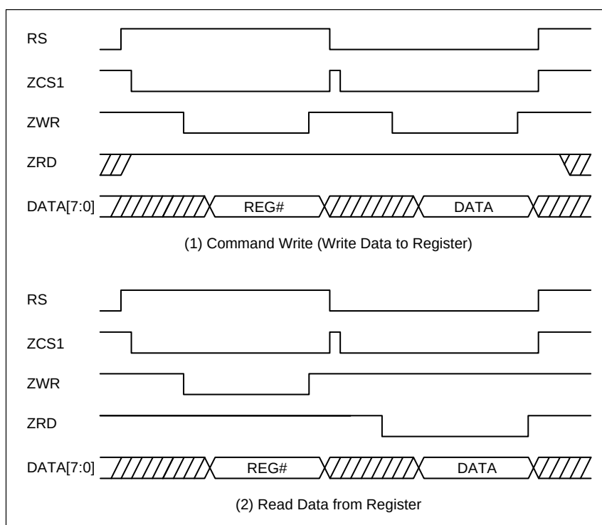
图 6-5：「写入指令」与「缓存器读取」
