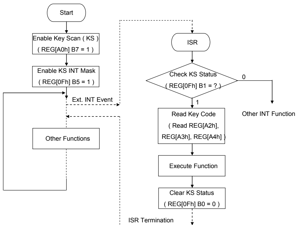
图 6-24 : 键盘扫描功能的流程图 (2)
