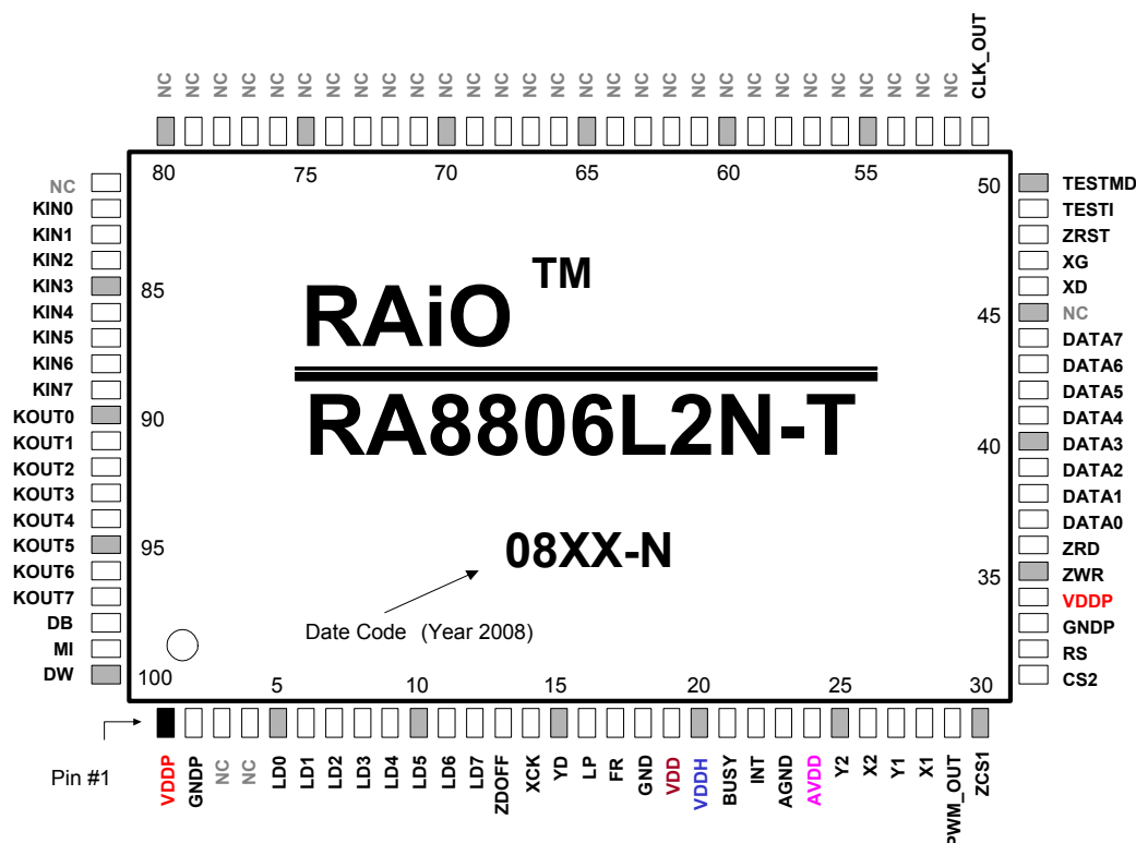
图 7-2 : LQFP-100Pin 脚位定义图
