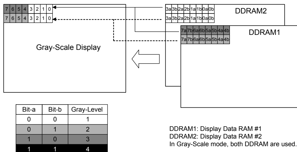
图 6-45 : 4 灰阶显示的对映方式
