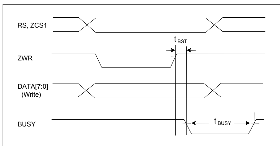
图 6-36 : BUSY 时序图
