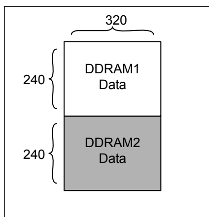
图 6-68 : 扩展模式 (2) 缓存器 MAMR Bit[6:4] = 111h
