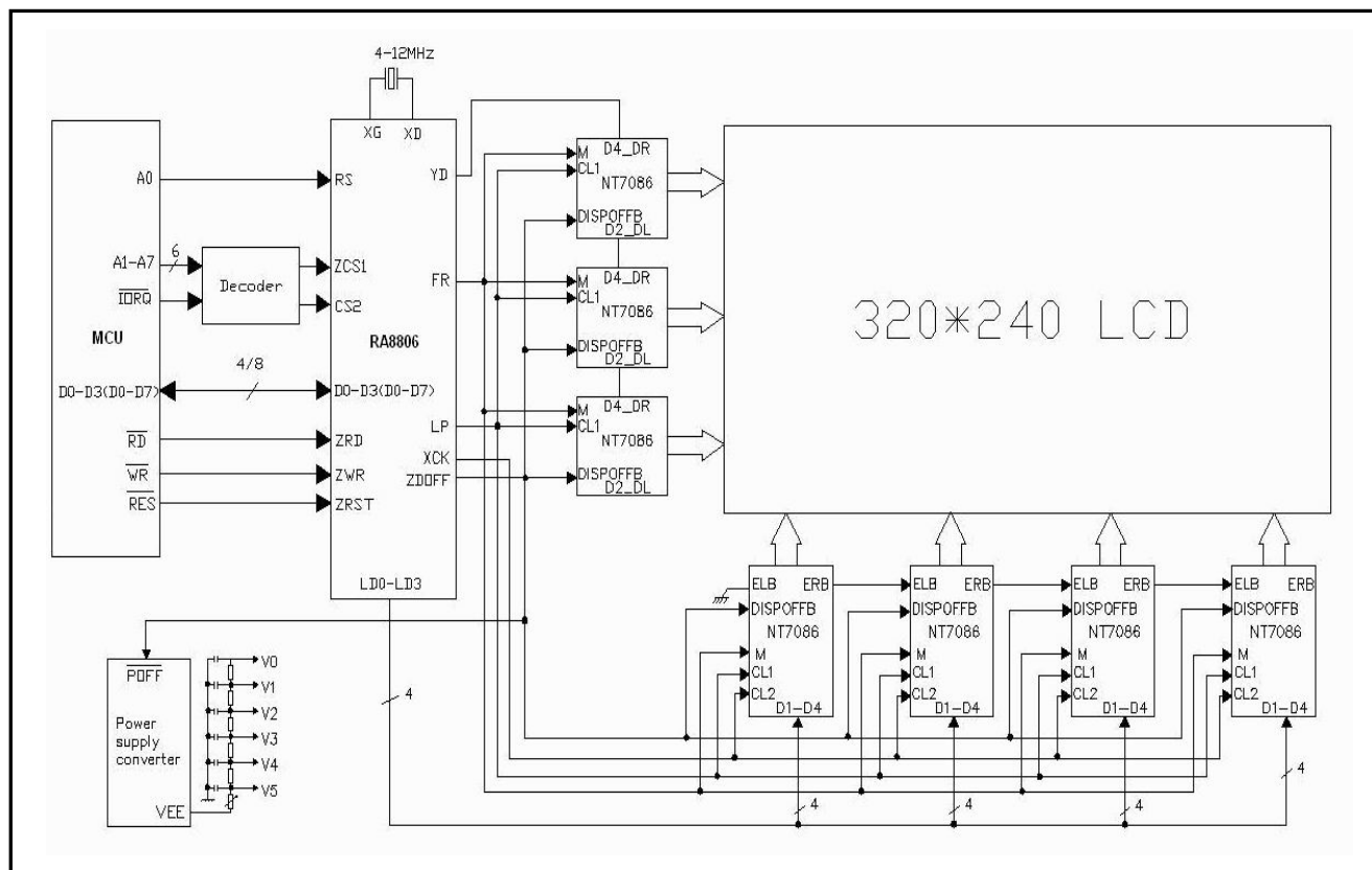
图 6-10 : 320x240 液晶显示屏的应用方块图
