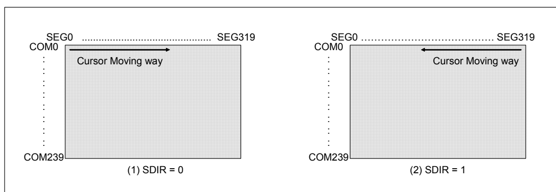
图 6-14 : 改变 Segment 显示顺序之范例
