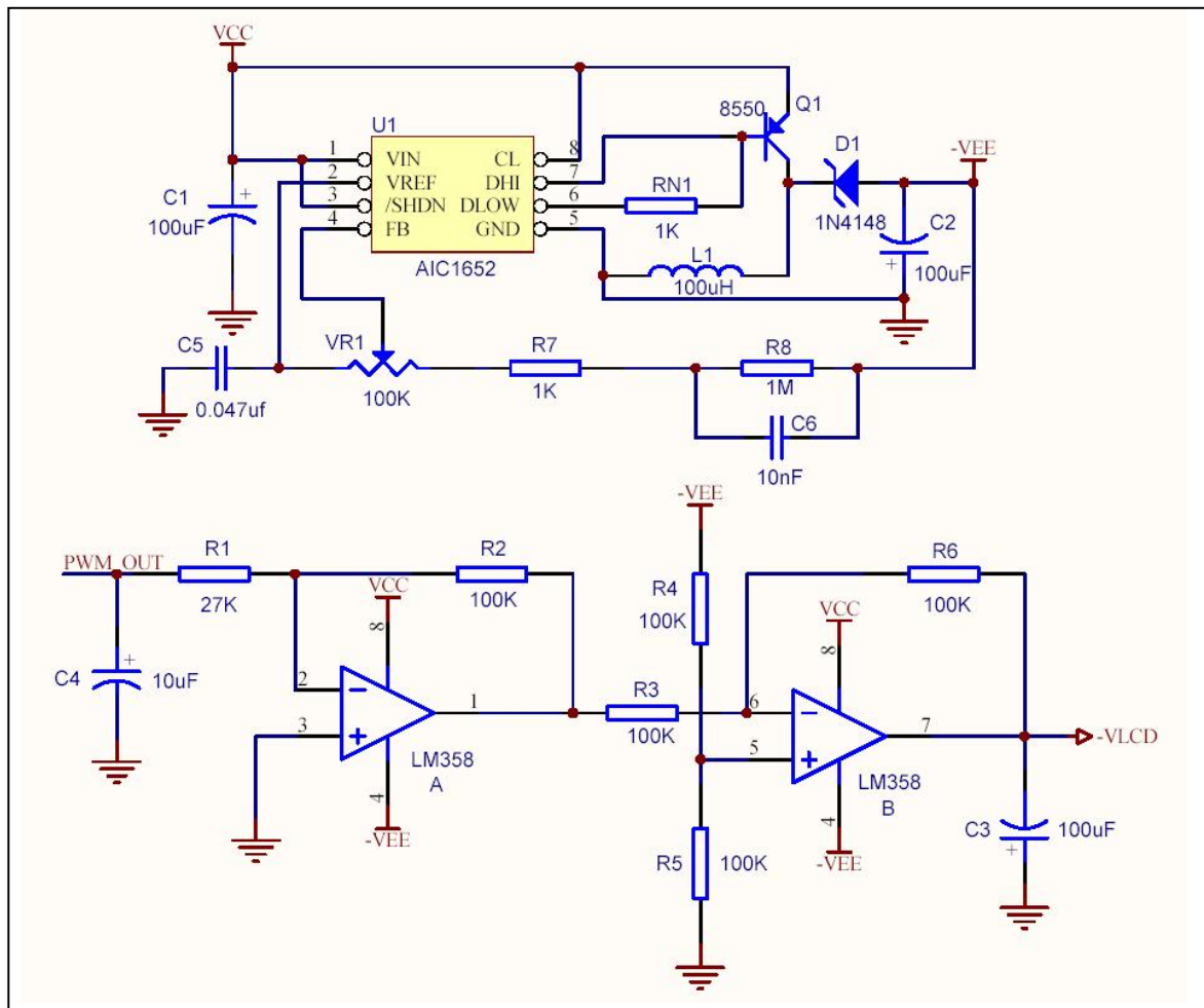
图 6-39 : PWM 控制负极性的 VLCD 的应用电路
