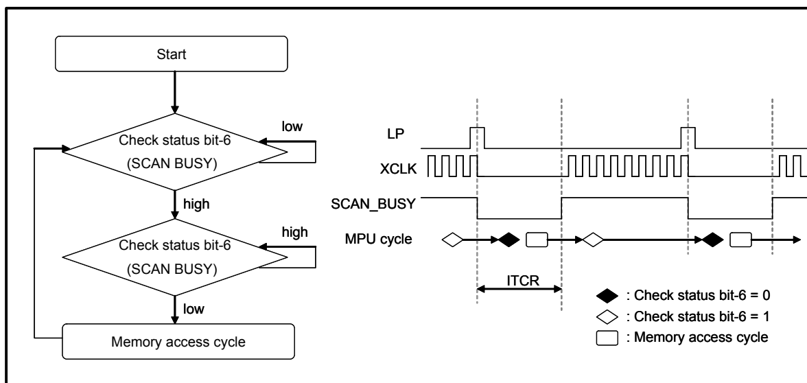
图 6-76 : 以 Check BUSY 来消除雪花的理想状况 (2)
