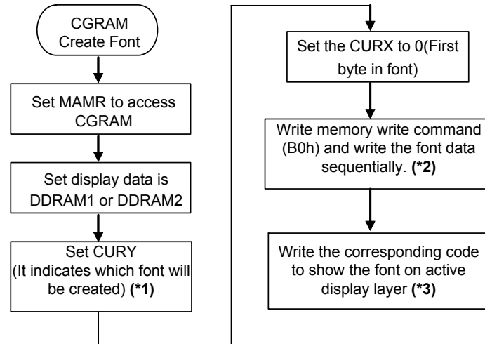
图 6-53 : 在 CGRAM 创造字型的流程图
