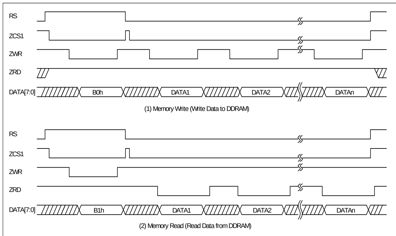
图 6-6 : 内存写入与读取
