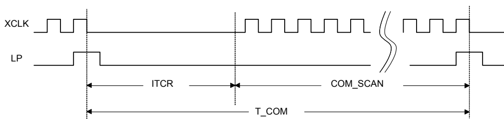
图 6-15 : LP 与 XCLK 信号之间的闲置时间
