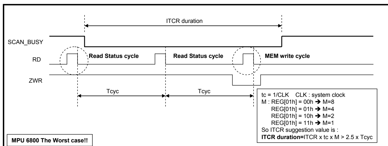
图 6-80 : MPU 6800 界面消除雪花 ITCR 建议值
