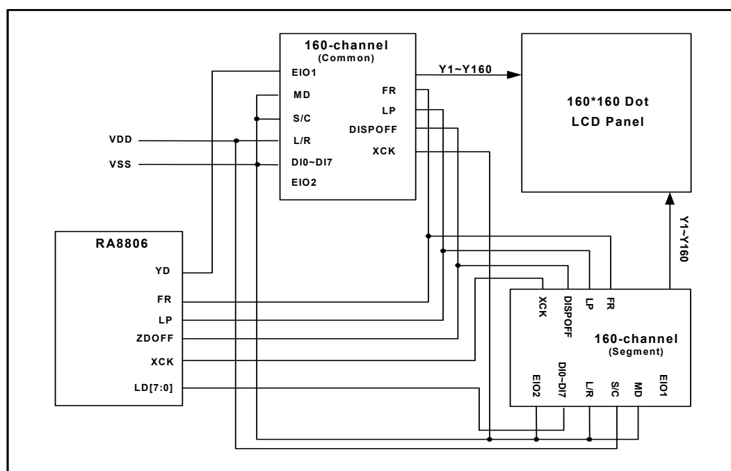
图 6-11 : 160x160 液晶显示屏的应用方块图
