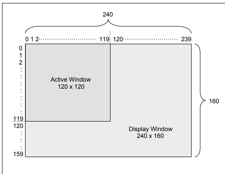
图 6-13 : RA8806 「显示窗口」与「工作窗口」
