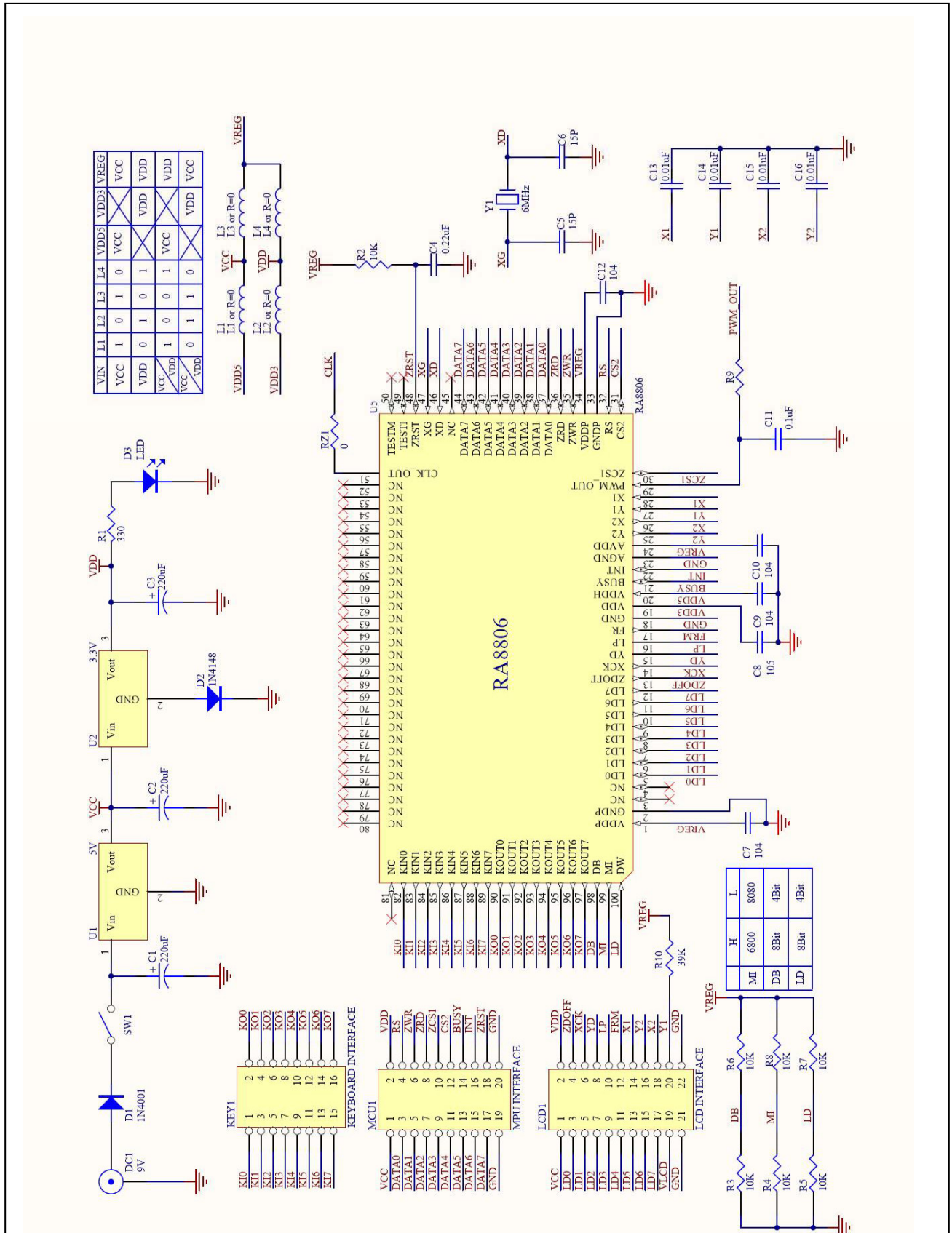
图 A-1: 3V 或 5V 之应用电路图
