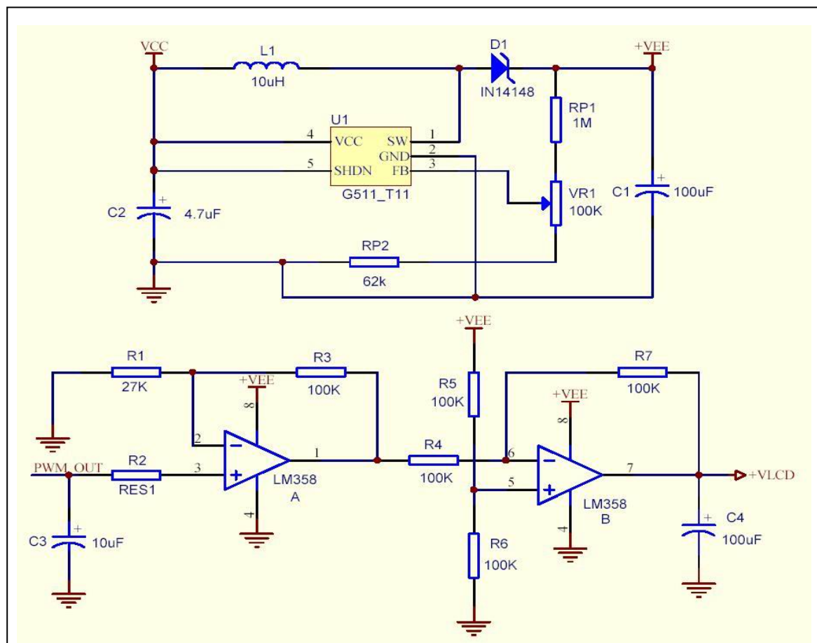
图 6-38 : PWM 控制正极性的 VLCD 的应用电路
