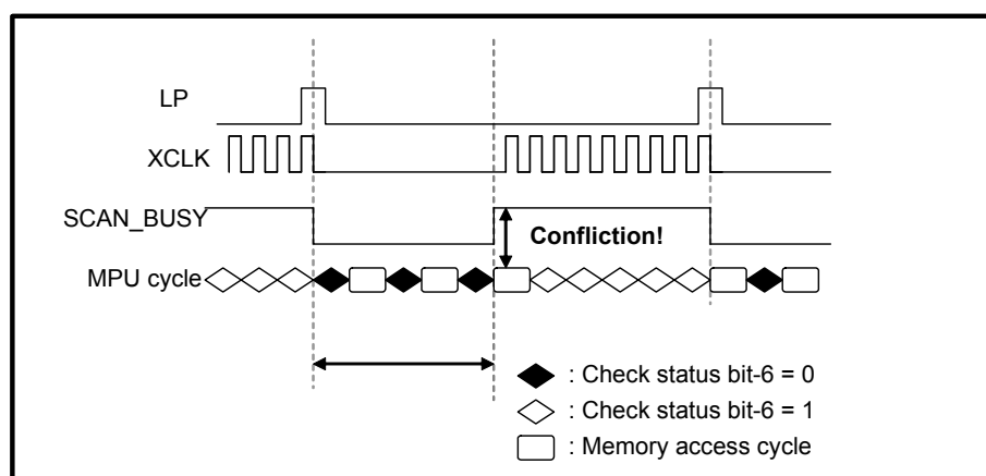
图 6-75 : 以 Check BUSY 来消除雪花的非理想状况 (1)
