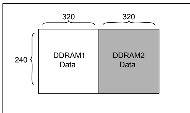
图 6-67 : 扩展模式（1）缓存器 MAMR Bit[6:4] = 110h
