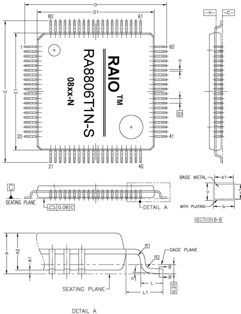
图 7-5 : TQFP-80Pin 机构图
