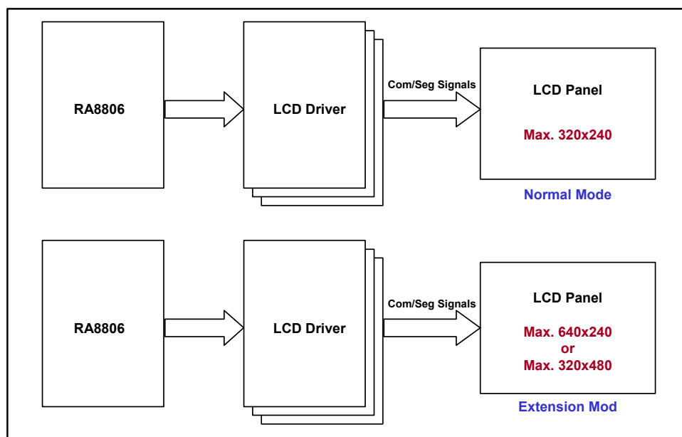
图 6-66 : RA8806 的最高显示点数
