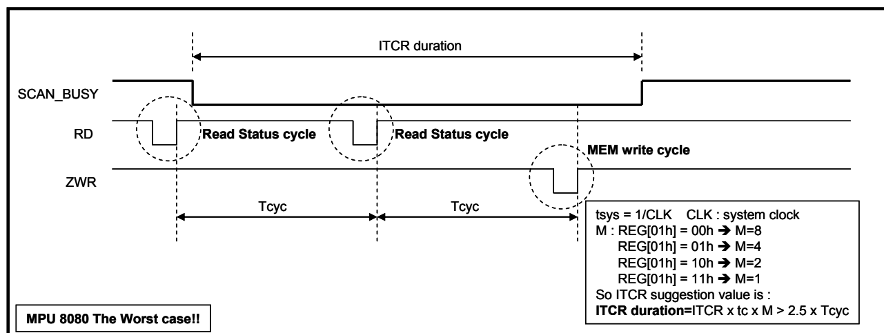
图 6-79 : MPU 8080 界面消除雪花 ITCR 建议值
