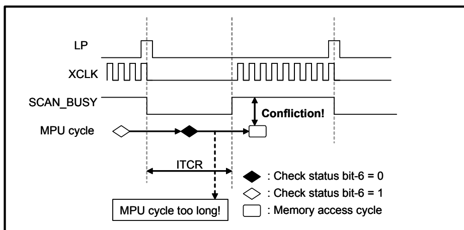
图 6-77 : MPU 周期过长造成以 Check BUSY 来消除雪花效果不理想 (2)
