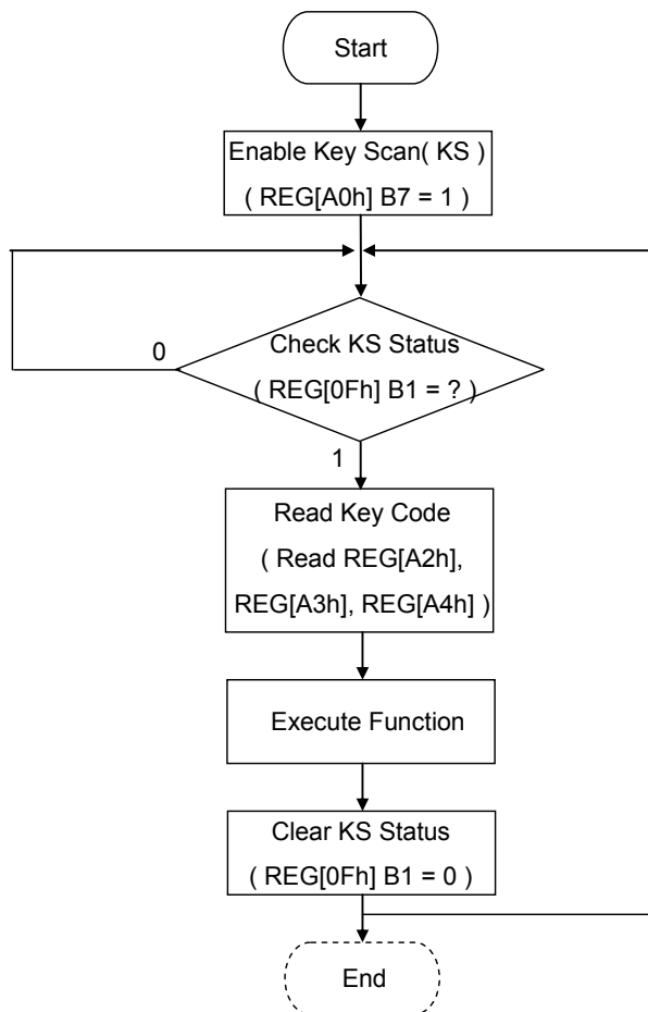
图 6-23 : 键盘扫描功能的流程图 (1)
