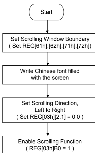
图 6-57：水平卷动流程图
