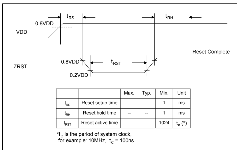
图 6-28: 重置时序参数
