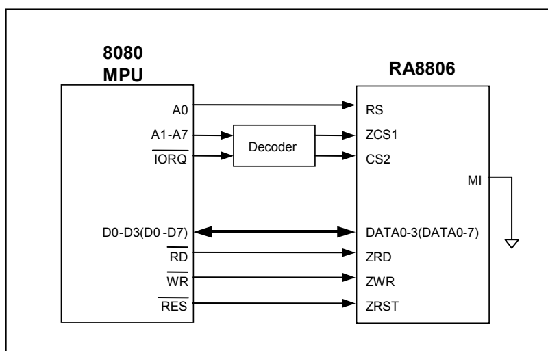
图 6-1 : 8080 (4/8-位) MPU 接口
