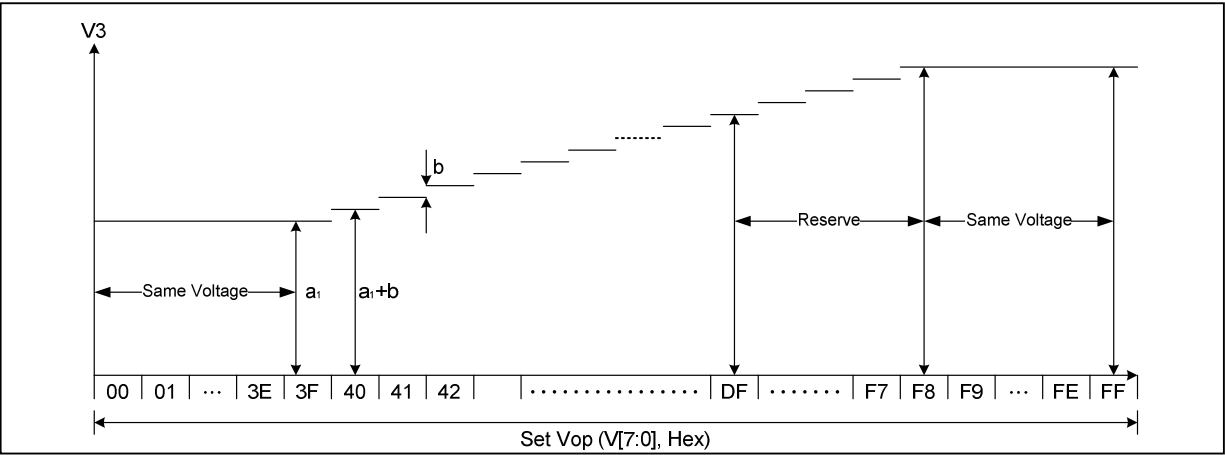
Fig 9. Setting V3 Voltage
