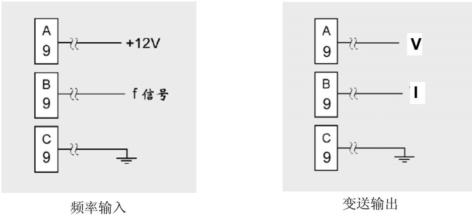
图 3-3-3 频率输入、变送输出接线图
