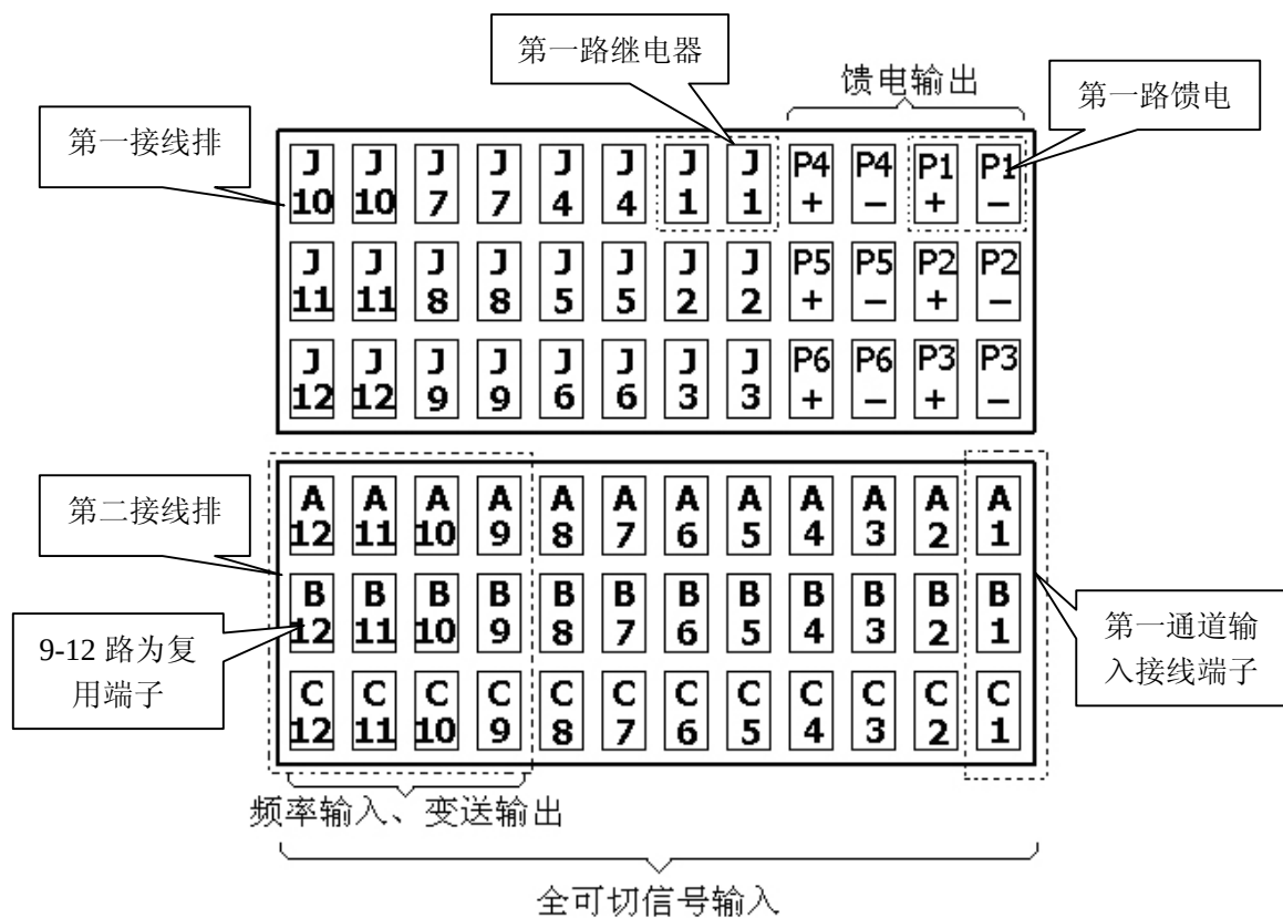
图 3-3-1-B 端子排列示意图
