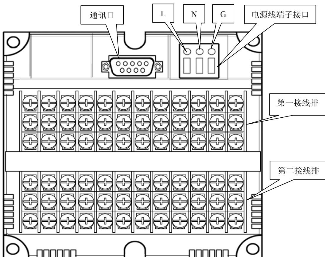
图 3-3-1-A 端子排列图
