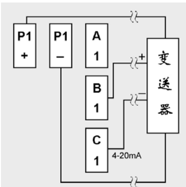
图 3-3-4 变送器接线图
