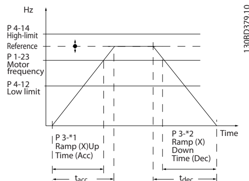
图 4.10 斜坡 1 示例
