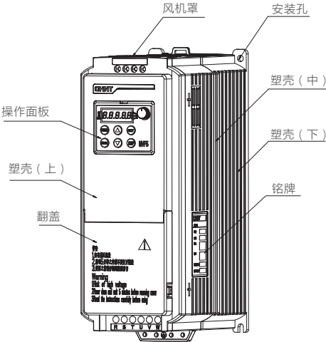
图5-3 NVF5-11/TS4-B ~ NVF5-22/TS4-B、NVF5-11GS ~ NVF5-22GS外形部件图
