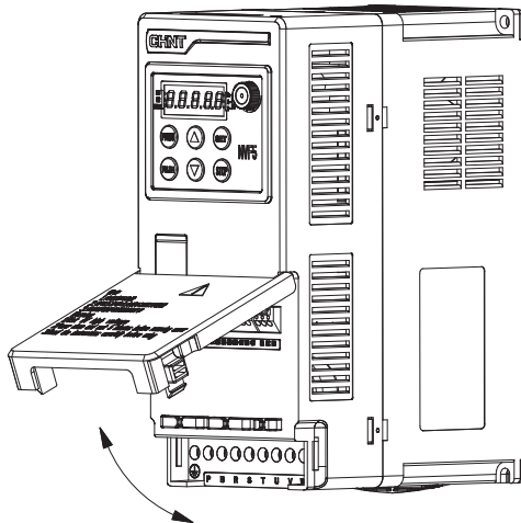
图7-4 NVF5-3.7/TS4-B~NVF5-7.5/TS4-B、NVF5-3.7GS~NVF5-7.5GS翻盖示意图
