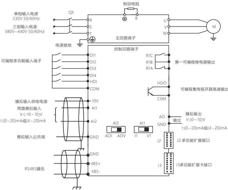
图5-5 NVF5-0.4TD2~NVF5-7.5/TS4端子的接线图
