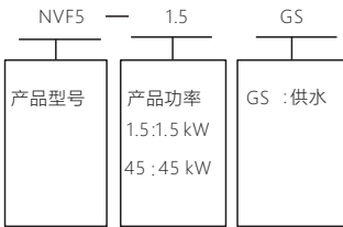
图2-4 NVF5-GS系列变频器产品型号命名规则
