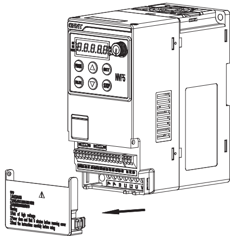
图7-3 NVF5-0.4/TD2~NVF5-2.2/TS4-B、NVF5-1.5GS NVF5-2.2GS翻盖示意图
