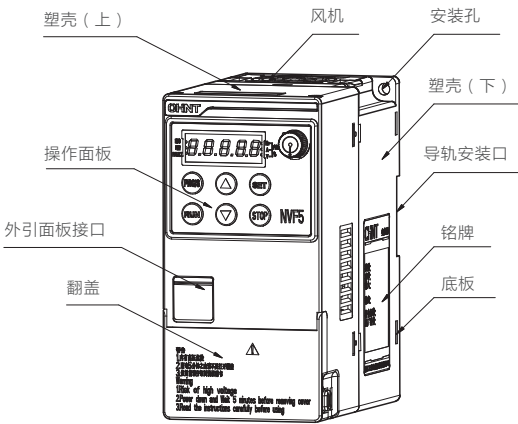
图5-1 NVF5-0.4/TD2 ~ NVF5-2.2/TD2和NVF5-0.4/TS4-B ~ NVF5-2.2/TS4-B、NVF5-1.5GS ~ NVF5-2.2GS外形部件图 (NVF5-2.2/TD2机型的风机安装在变频器的底部)
