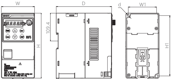
图6-1 NVF5-0.4/TD2 ~ NVF5-2.2/TD2和NVF5-0.4/TS4-B ~ NVF5-2.2/TS4-B、NVF5-1.5GS ~ NVF5-2.2GS 外形与安装尺寸图
