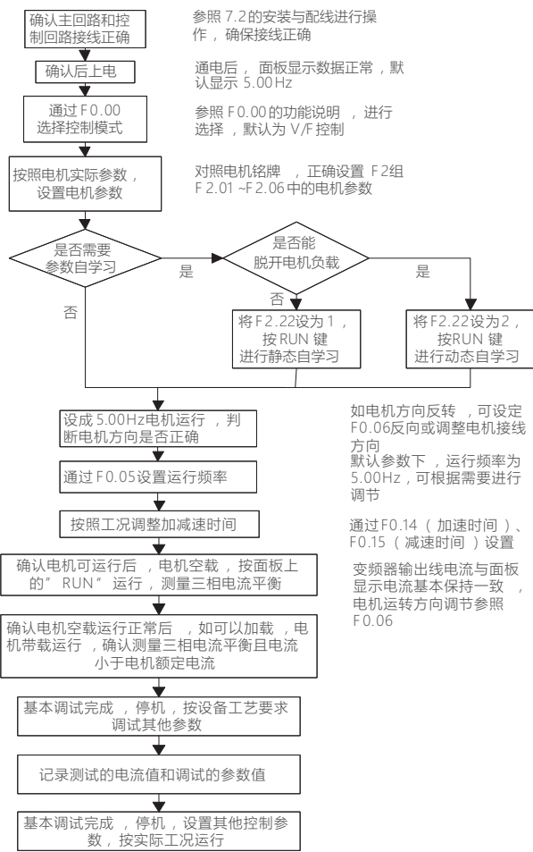
图7-16 基本调试操作图
