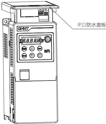
图7-2 安装IP22防护盖板外形图
