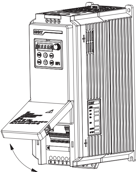
图7-5 NVF5-11/TS4-B~NVF5-11GS~NVF5-22GS翻盖示意图
