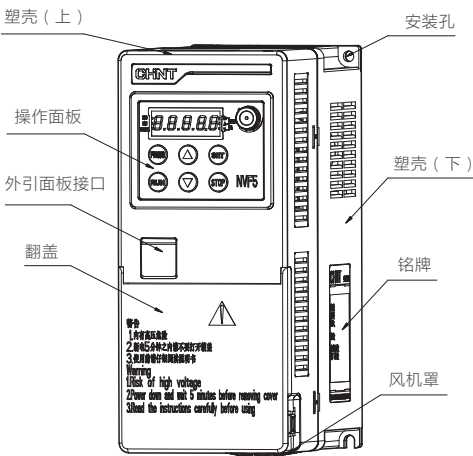
图5-2 NVF5-3.7/TS4-B ~ NVF5-7.5 /TS4-B、NVF5-3.7GS ~ NVF5-7.5GS外形部件图
