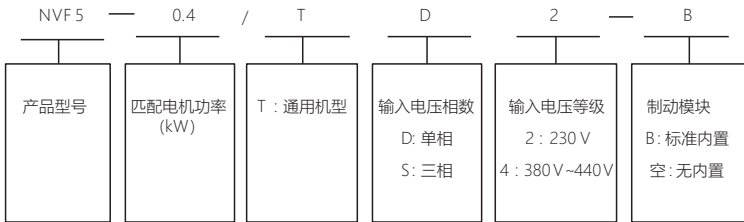
图2-3 NVF5系列变频器产品型号命名规则
