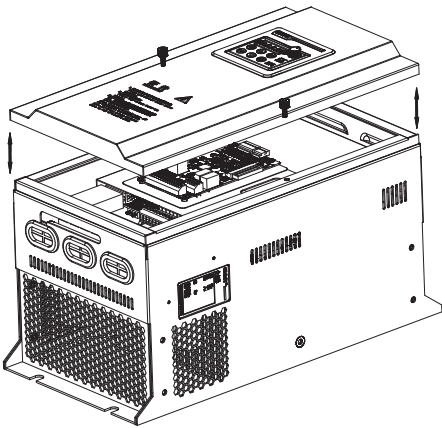
图7-6 NVF5-30GS~NVF5-45GS 上盖示意图
