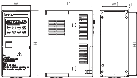
图6-2 NVF5-3.7/TS4-B ~ NVF5-7.5/TS4-B、NVF5-3.7GS ~ NVF5-7.5GS外形与安装尺寸图
