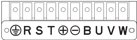
图5-11 主回路端子NVF5-30GS
