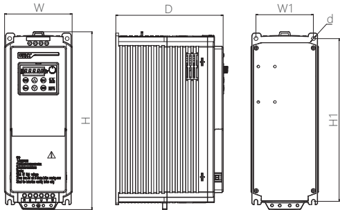
图6-3 NVF5-11/TS4-B ~ NVF5-22/TS4-B、NVF5-11GS ~ NVF5-22GS外形与安装尺寸图
