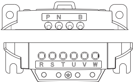
图5-10 主回路端子NVF5-11/TS4-B~22/TS4-B、NVF5-11GS~22GS
