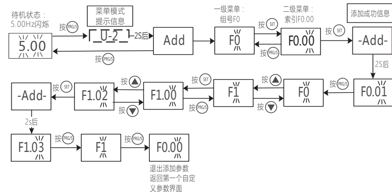
图7-13 自定义菜单模式首次添加参数
