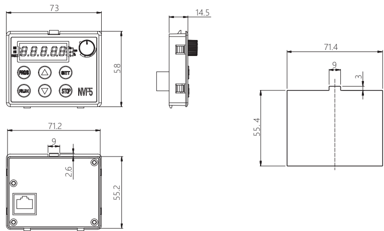
图6-5 显示面板尺寸图
