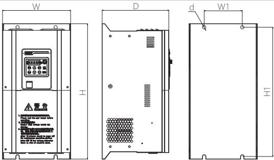
图6-4 NVF5-30GS ~ NVF5-45GS外形与安装尺寸图
