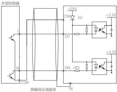
图5-15 使用变频器内部+24V电源的源极连接方式
