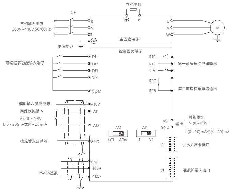
图5-6 NVF5-1.5GS~NVF5-7.5GS端子的接线图
