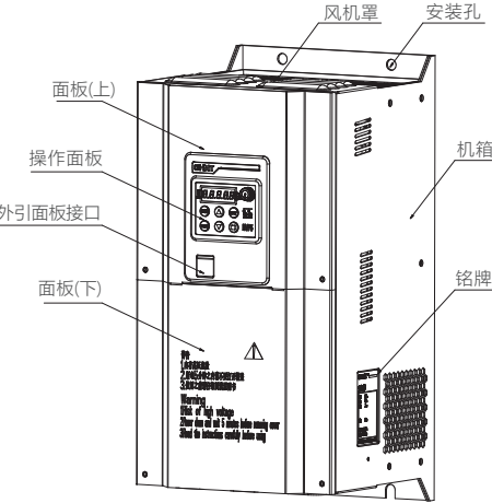
图5-4 NVF5-30GS ~ NVF5-45GS 外形部件图
