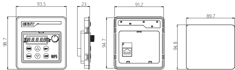
图6-7 托板外形尺寸图
