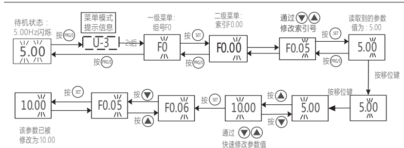
图7-15 工程型菜单参数设定
