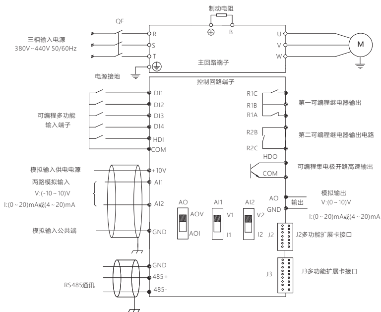
图5-7 NVF5-11/TS4~NVF5-22/TS4、NVF5-11GS~NVF5-45GS端子的接线图
