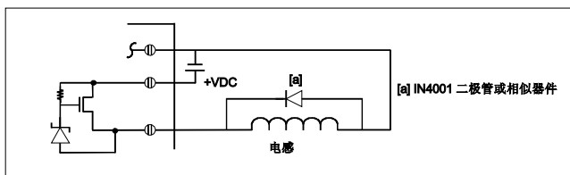
直流晶体管输出的普通二极管抑制
