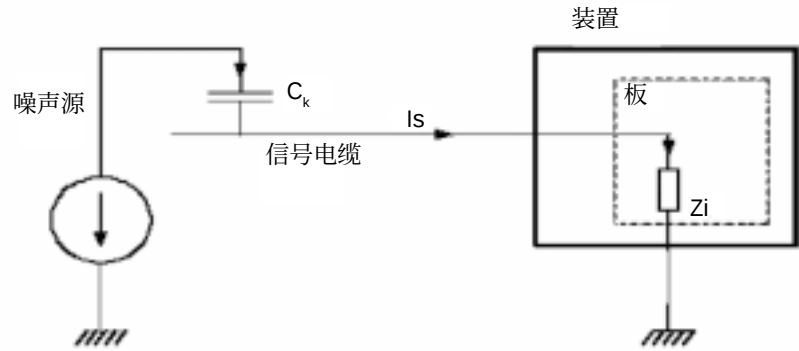
无屏蔽信号电缆的耦合电容
