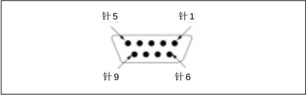
S7-200 CPU 通讯口引脚分配
