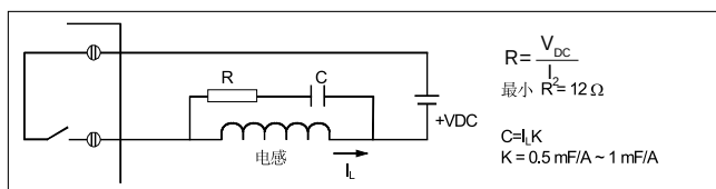
图中继电器驱动 DC 负载上跨接电阻电容网络保护电路
