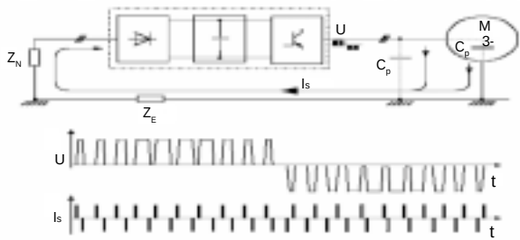
变频器输出电压 U 和噪声电流 I_s 的波形图
