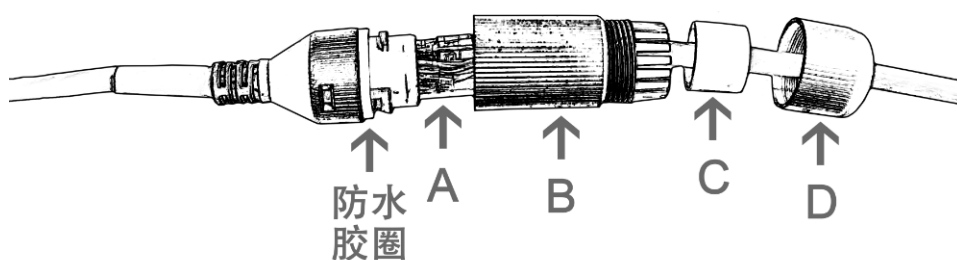
图 3-7 网线穿过防水堵头
