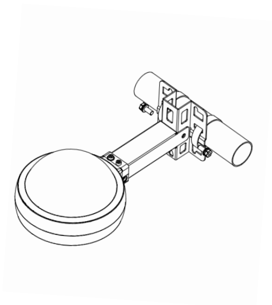
图 3-6 水平抱杆安装方式
