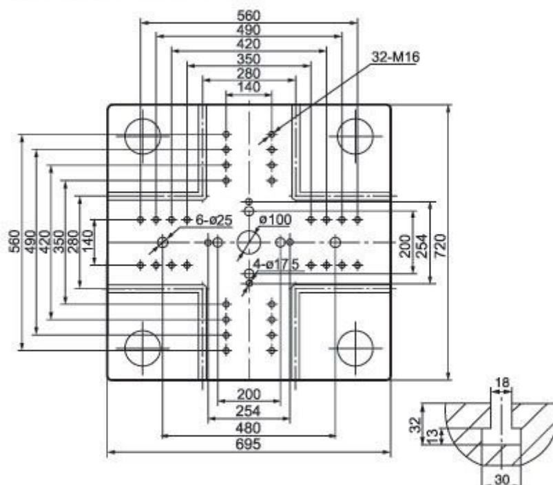
Platen dimensions 模板正面尺寸
