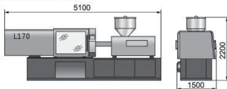
Dimension 外形尺寸
