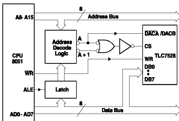
图5 TLC7528-Intel 8051接口
