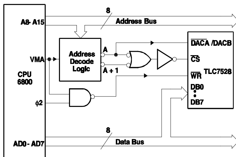
图6 TLC7528-6800接口
