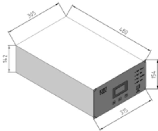
图 2-3 控制器简图
