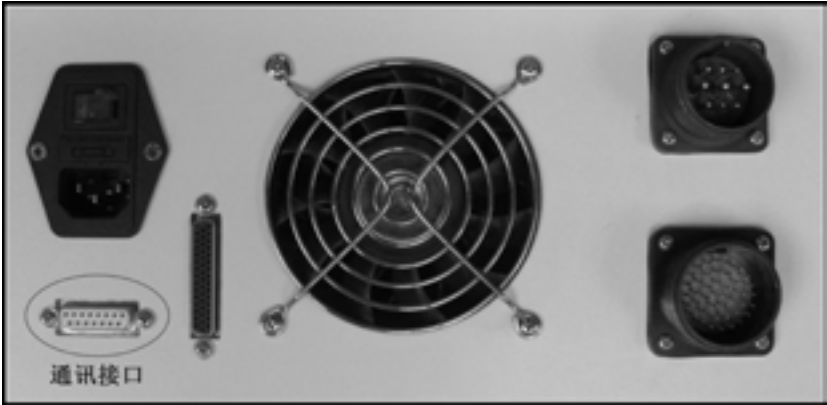
图 3-9 通讯接口位置示意图
