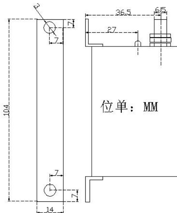
JZ882 接口示意图
