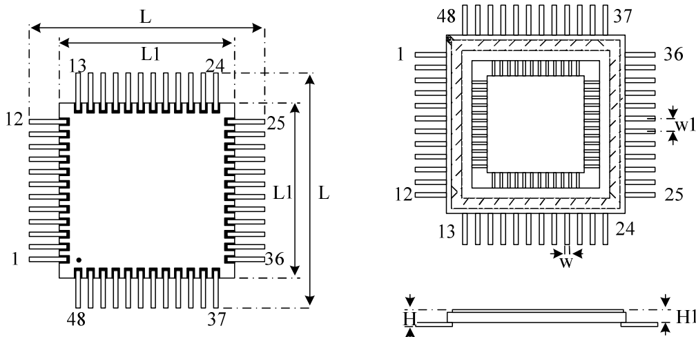
图 3 CS7123 外形图
