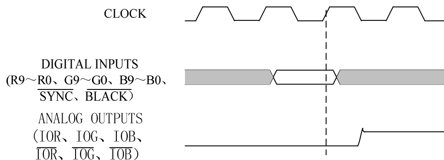
图 4 CS7123 时序图
