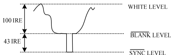
图 5 RGB 视频输出波形
