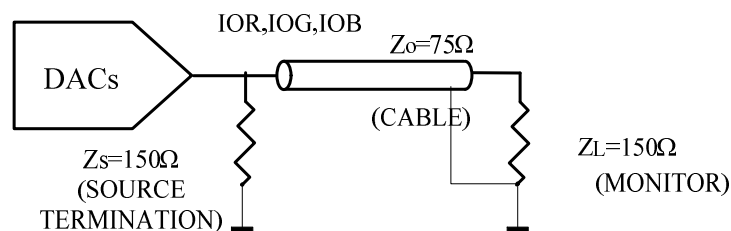
图6 针对 RS-343A 的模拟输入终端
