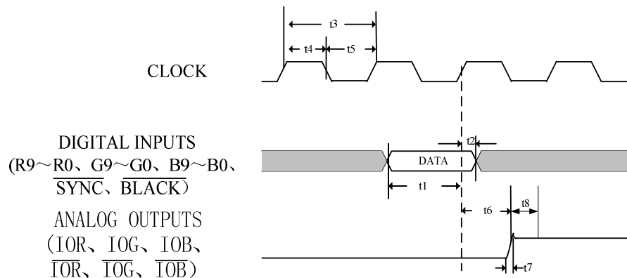
图 1. 时序图
