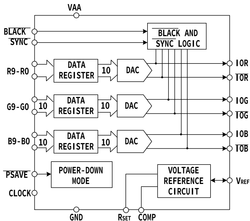
图 1 CS7123 功能框图
