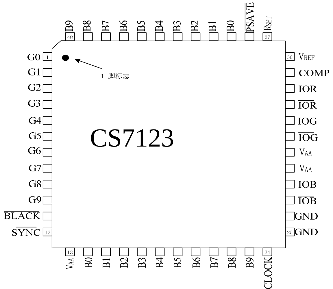
图 2 CS7123 管脚图
