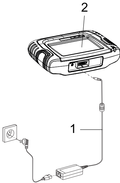
图. 4: 自检连接
