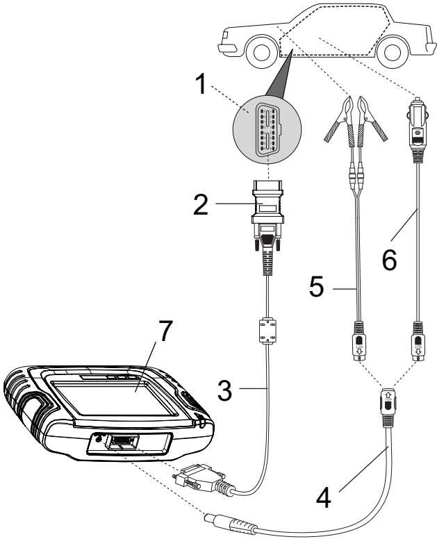
图. 3: 诊断连接
