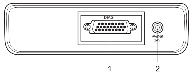
图. 1: 诊断端口
