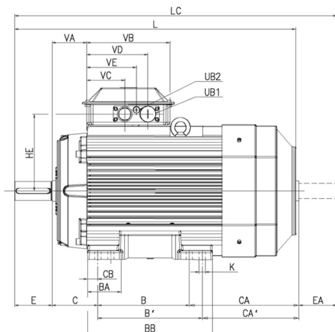
IM B3 (IM 1001), IM 1002
