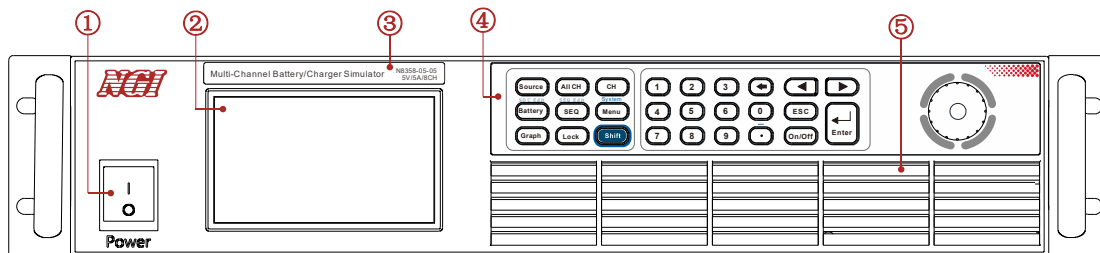
图 3-4 前面板
