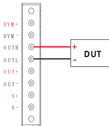
图 3-14 两线本地测量
