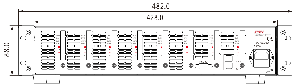
图 3-3 后面板尺寸
