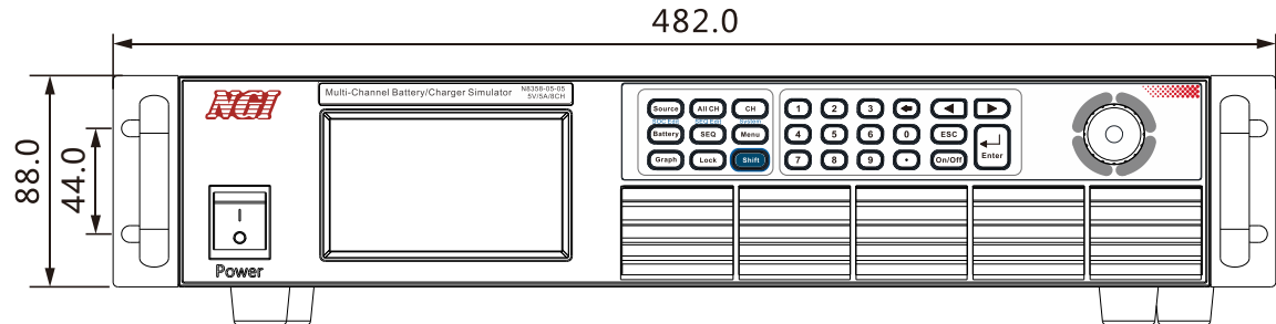
图 3-1 前面板尺寸
