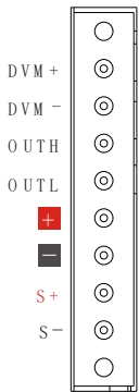
图 3-11 通道端口/DVM 输入端口
