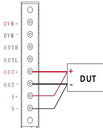
图 3-15 四线远端测量
