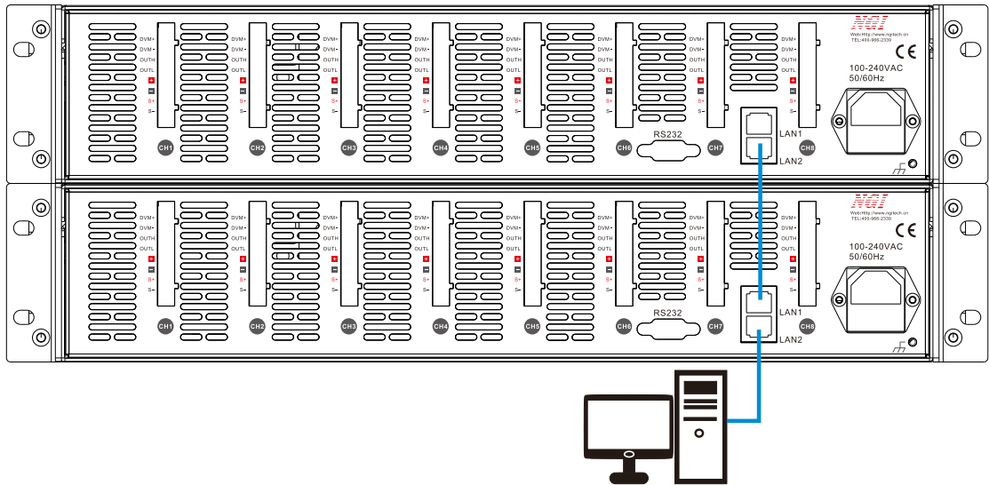
图 3-13 多机控制接线图
