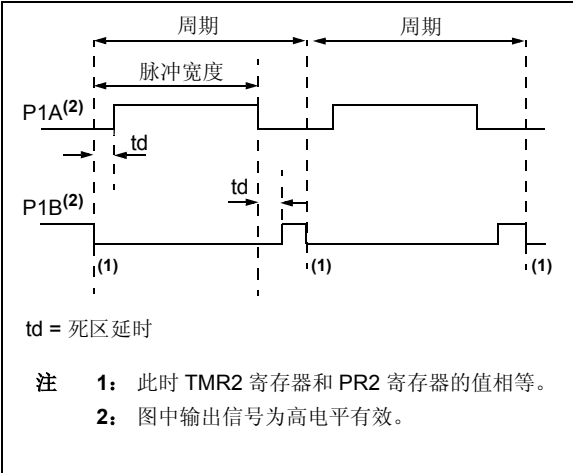
图 10-16: 半桥 PWM 输出示例
