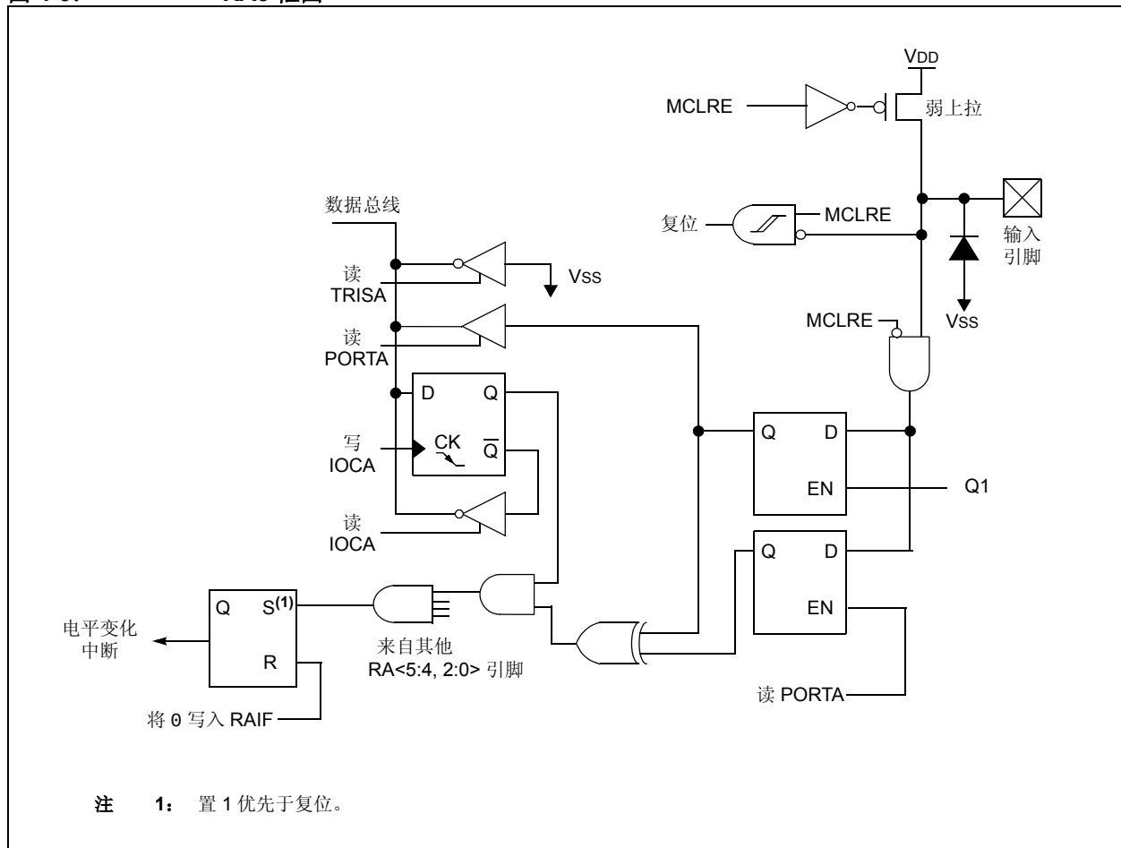
图 4-3: RA3 框图
