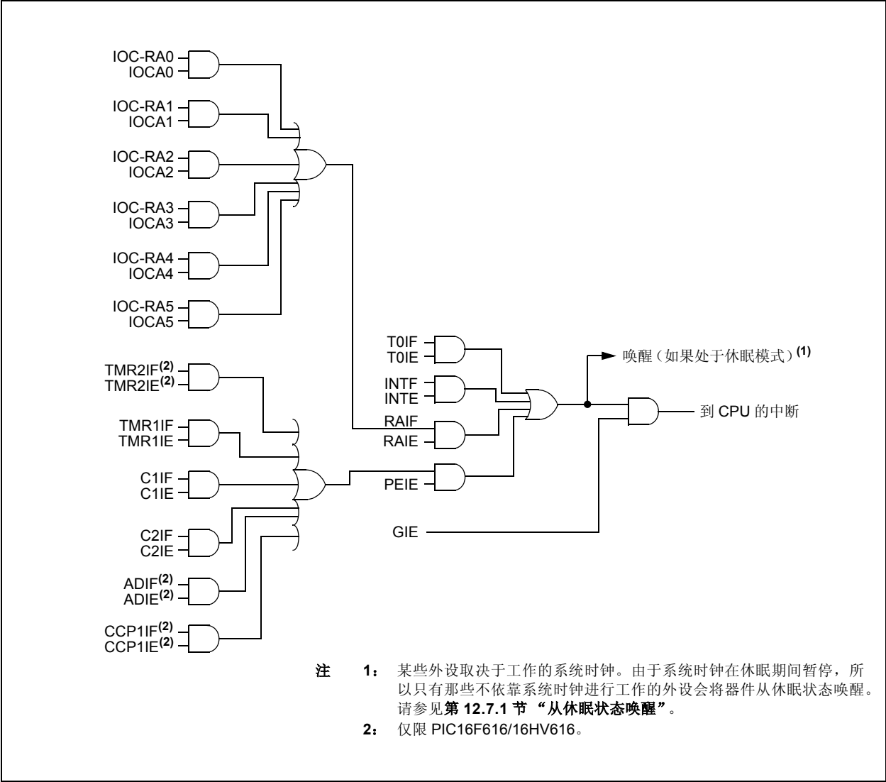
图 12-7: 中断逻辑
