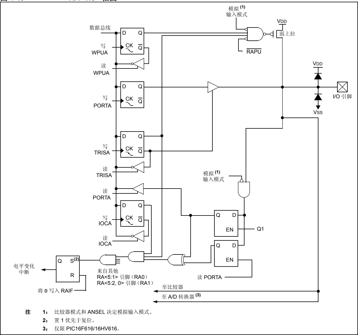
图 4-1: RA<1:0> 框图
