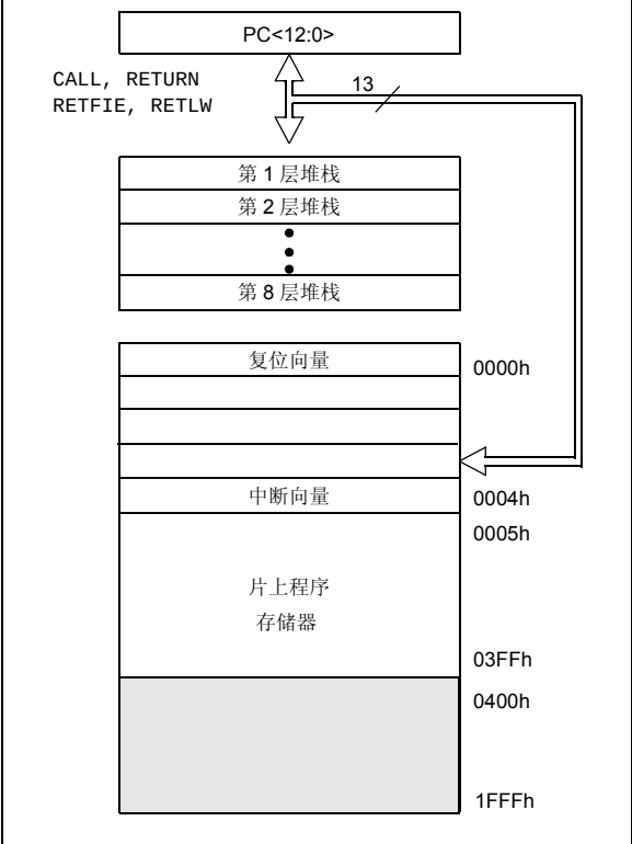
图 2-1: PIC16F610/16HV610 的程序存储器映射和堆栈
