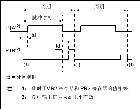
图 10-8: 半桥 PWM 输出示例
