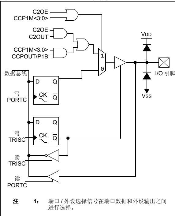
图 4-8: RC4 框图
