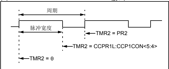
图 10-4: CCP PWM 输出
