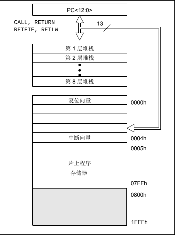
图 2-2: PIC16F616/16HV616 的程序存储器映射和堆栈
