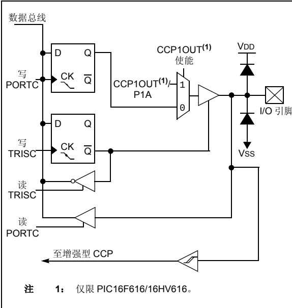
图 4-9: RC5 引脚框图
