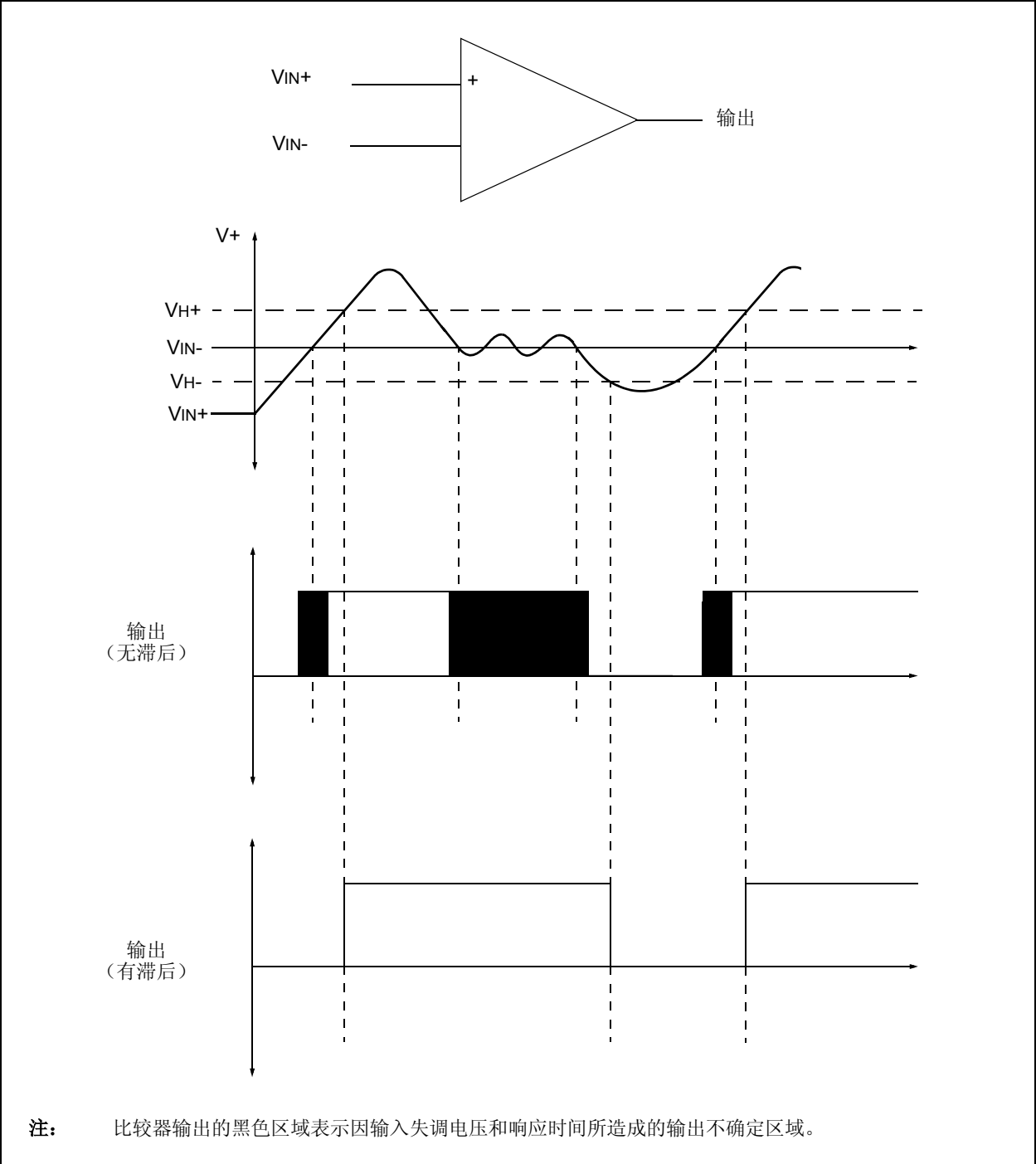
图 8-7: 比较器滞后
