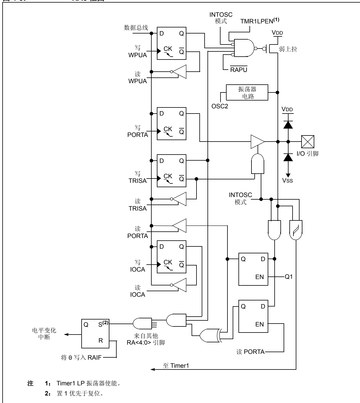
图 4-5: RA5 框图
