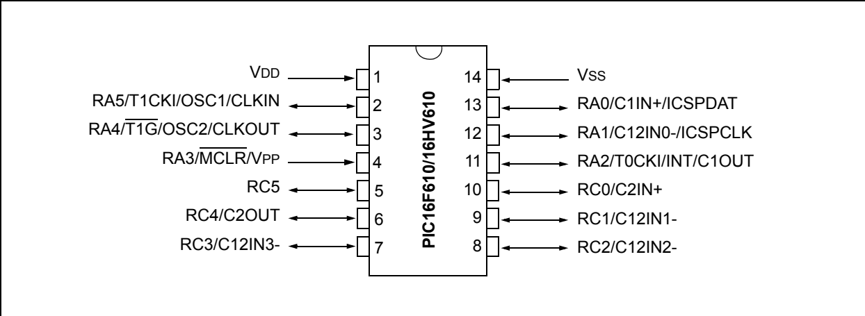
PIC16F610/16HV610 14 引脚示意图 (PDIP、SOIC 和 TSSOP)
