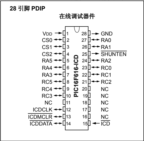
图 12-11: 28 引脚 ICD 引脚排列
