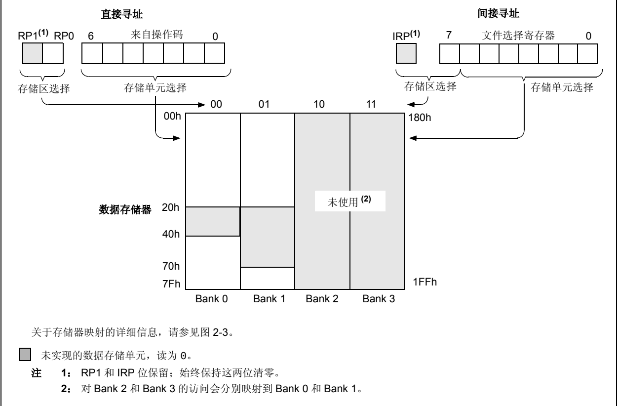
图 2-6: PIC16F610/16HV610 的直接 / 间接寻址
