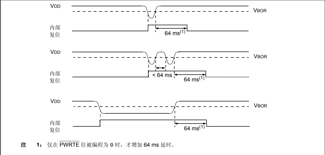
图 12-3: 欠压情形
