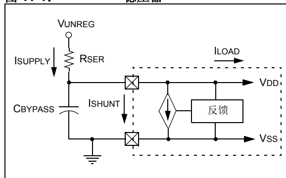
图 11-1: 稳压器
