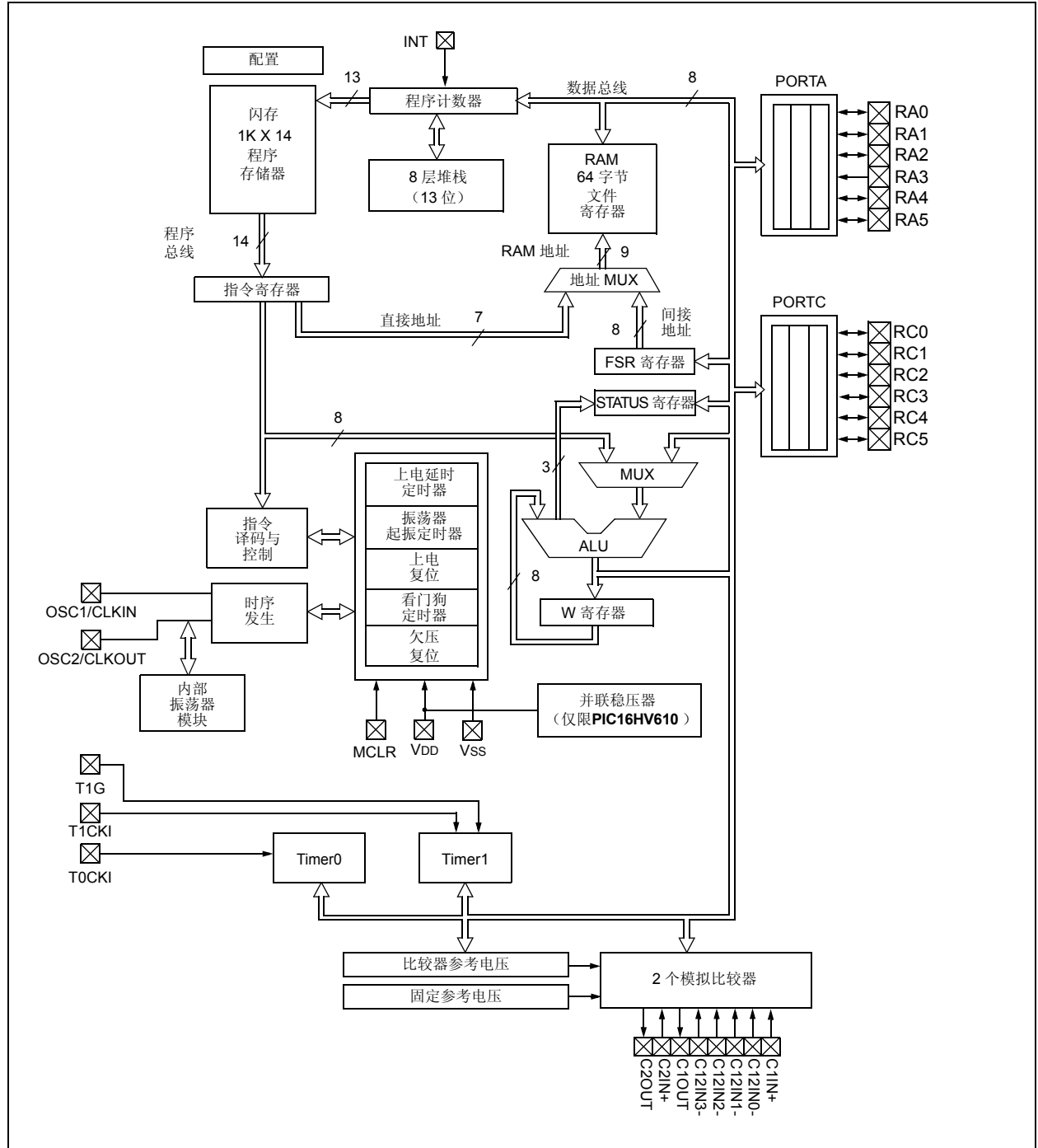
图 1-1: PIC16F610/16HV610 框图
