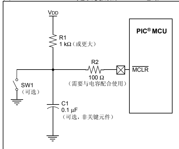
图 12-2: 建议使用的 \overline{MCLR} 电路
