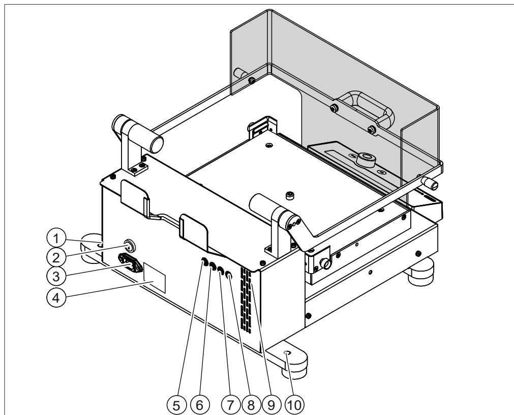
图 4: 后视图
