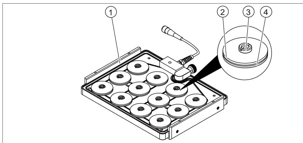
图 6: 盖底部
