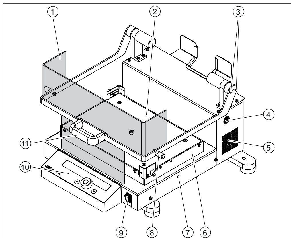
图 3: 前视图
