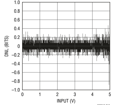
ADC 微分非线性
