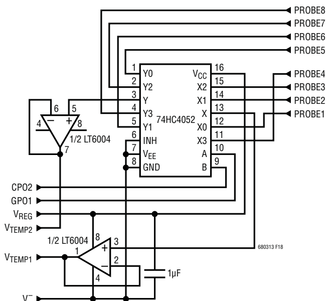
图 18：利用多路复用扩充传感器数目
