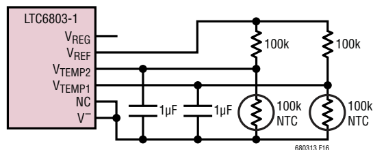
图 16：直接利用 V_{REF} 驱动热敏电阻
