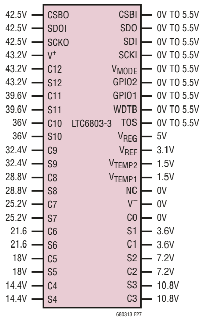
图 27：采用 12 节 3.6V 电池时的典型引脚电压
