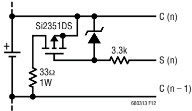
图 12：外部放电 FET 连接 (示出了一节电池)
