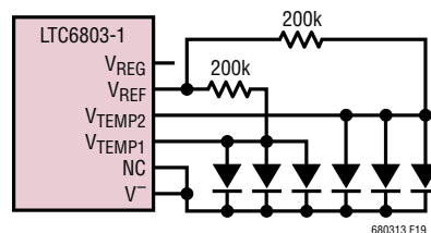
图 19：将二极管传感器用作热点探测器
