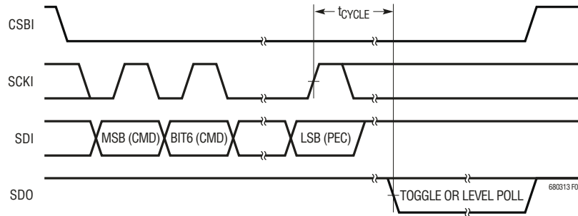
图 6：传输格式 (ADC 转换与轮询)
