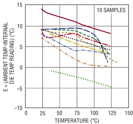
内部芯片温度测量误差 (采用一个 8mV/°K 比例因子)
