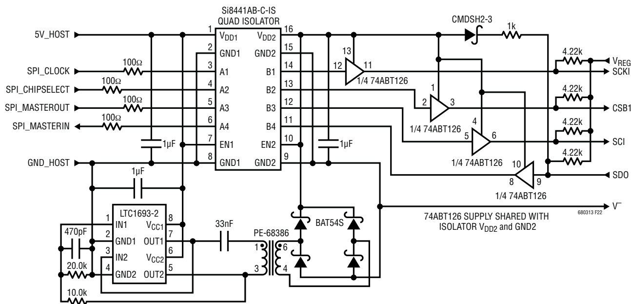
图 22：提供一个隔离式高速数据接口
