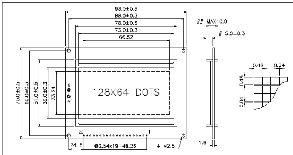
外形尺寸图
