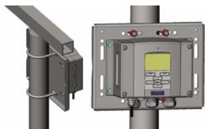
在杆/柱上安装用套件 用安装套件进行杆或管道 安装
