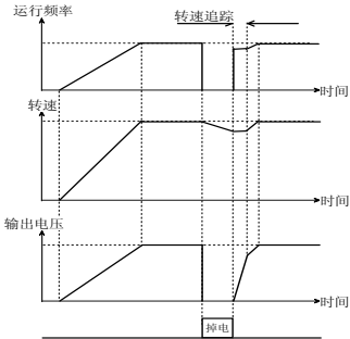
图 5-1-2 转速追踪
