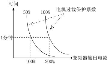
图 5-13-1 电机过载保护系数设定
