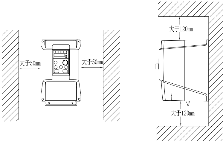
图 2-1 安装方向和空间
