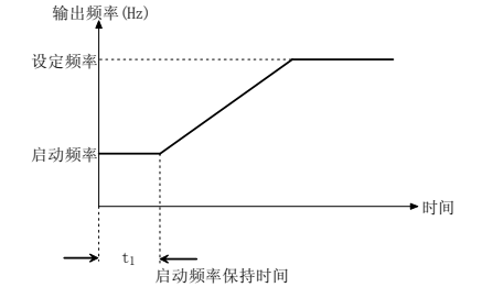
图 5-1-3 启动频率与启动时间示意图
