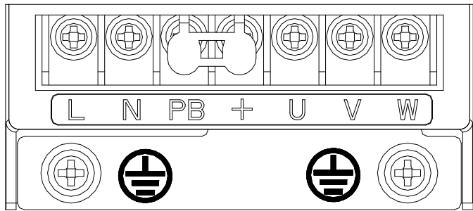
图 2-2 1PH 220V 0.4&0.75kW 主回路端子接线
