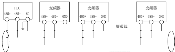
图 2-10 PLC与变频器多机通讯时推荐的接线图（变频器、电机全部良好接地）
