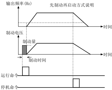
图 5-1-1 启动制动
