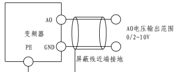
图 2-8 模拟输出端子配线图
