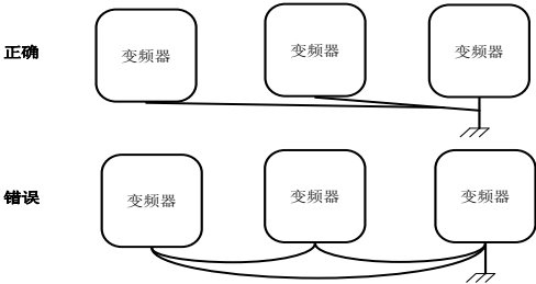
图 2-5 接地线连接方法
