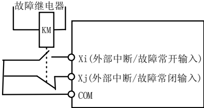
图 5-3-6 常开/常闭
