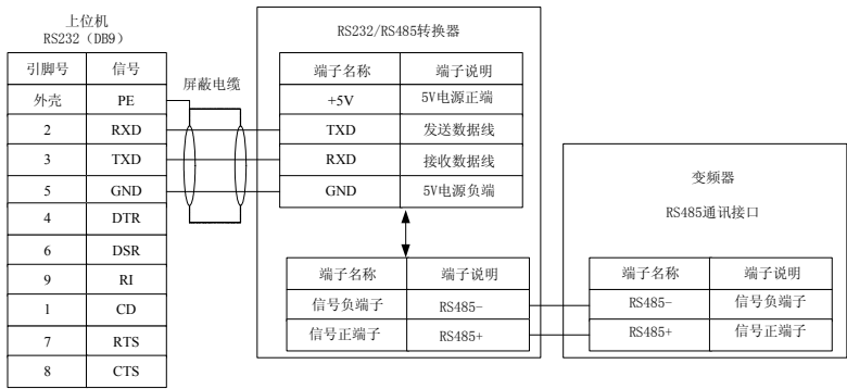
图 2-9 上位机与变频器接口接线图
