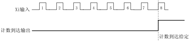
图 5-3-12 计数到达
