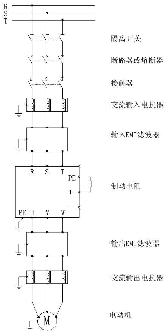
图 7-1 S2R4GB-3015GB 外围设备连接图
