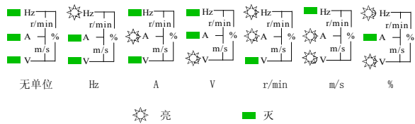
图 3-2 单位指示灯状态与单位对应关系图
