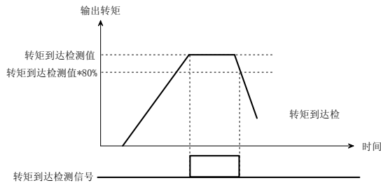
图 5-3-11 转矩到达检测
