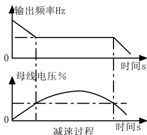
图 5-13-5 减速过程
