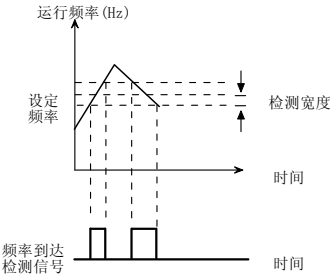
图 5-3-8 频率到达检测
