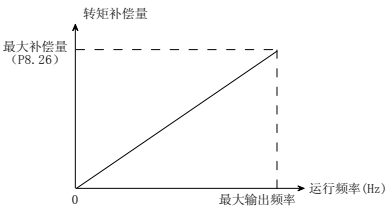
图 5-8-2 高速转矩补偿量与输出频率关系图
