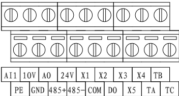
图 2-6 控制回路端子排布
