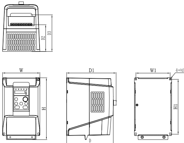
图 A1-1 外形示意图
