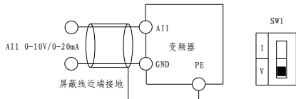
图 2-7 模拟输入端子配线图
