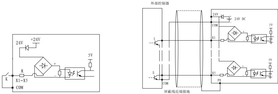
图2-11输入多功能端子配线连接图
