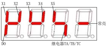
图 5-12-1 端子状态指示
