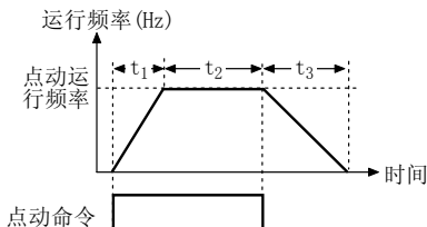
图 5-2-1 点动运行参数说明
