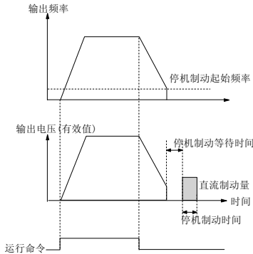
图 5-1-7 停机制动
