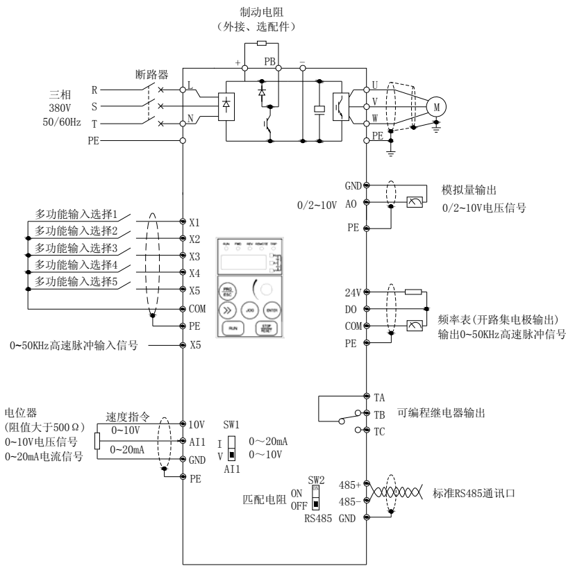
图 2-14 接线图
