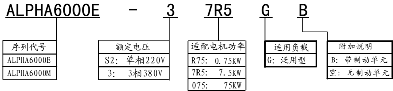
图 1-1 型号说明
