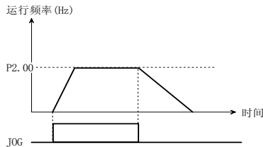
图 5-3-2 JOG运行
