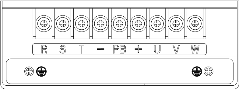
图 2-4 3PH 380V 4-30kW 主回路端子接线
