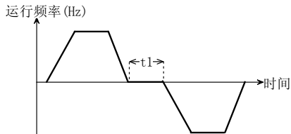
图 5-2-2 正反转切换时间
