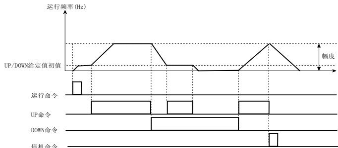
图 5-3-4 UP/DOWN 端子非组合运行
