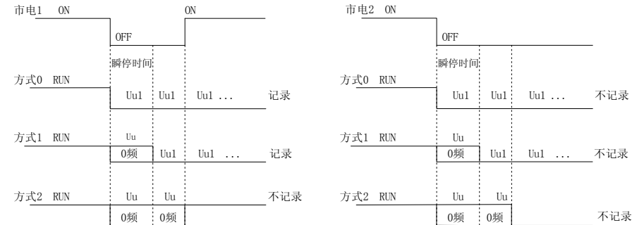
图 5-1-8 瞬停处理
