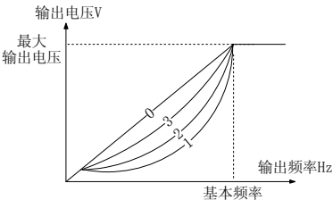
图 5-9-1 降转矩曲线
