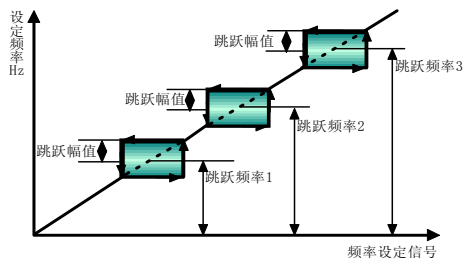
图 5-2-5 跳跃频率
