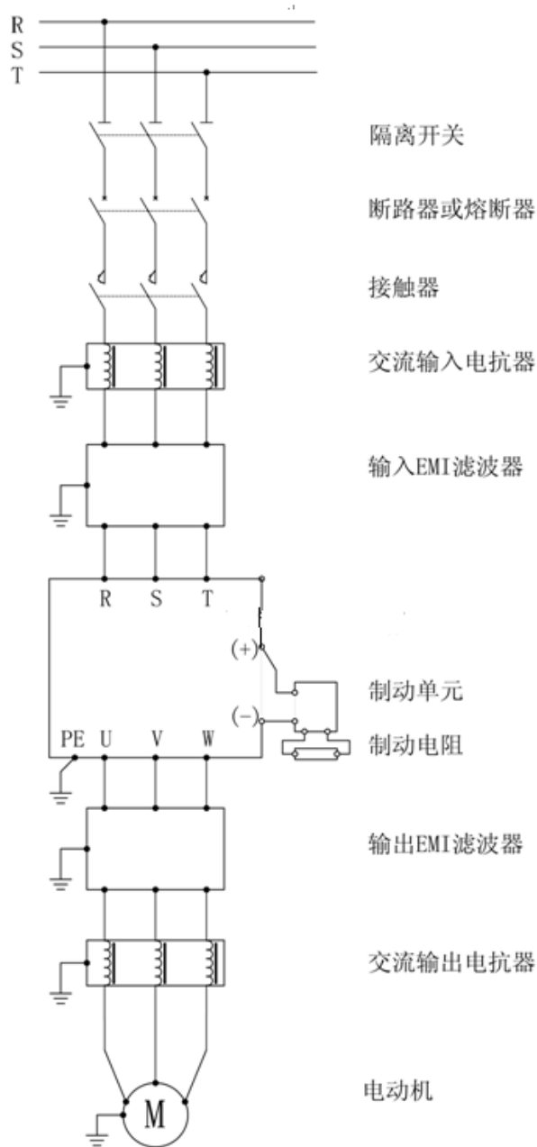
图 7-2 3018G-3030G 外围设备连接图
