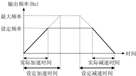
图 5-1-5 直线加减速
