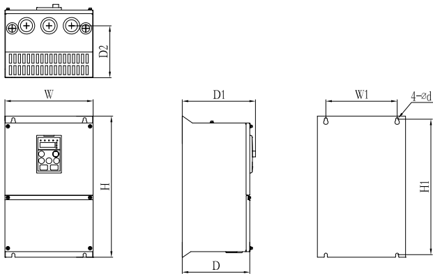
图 A1-2 外形示意图
