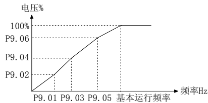
图 5-9-2 用户设定V/F曲线一般形式
