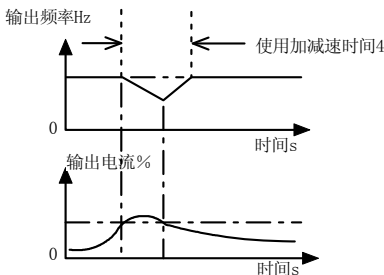
5-13-4 稳定运行过程
