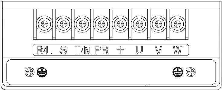
图 2-3 1PH 220V 1.5&2.2kW、3PH 380V 0.75-2.2kW 主回路端子接线
