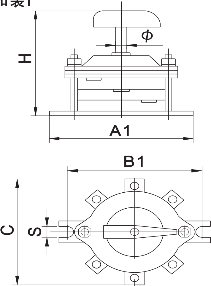
图A 板前接线式
