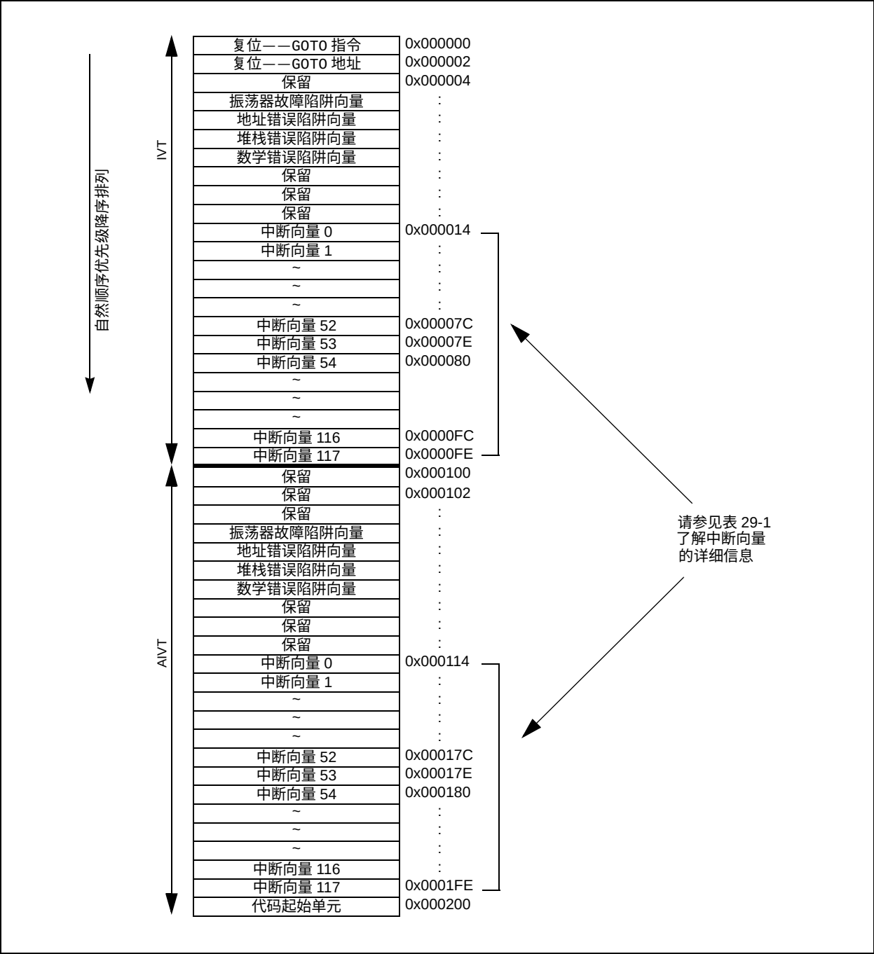
图 29-1： 中断向量表
