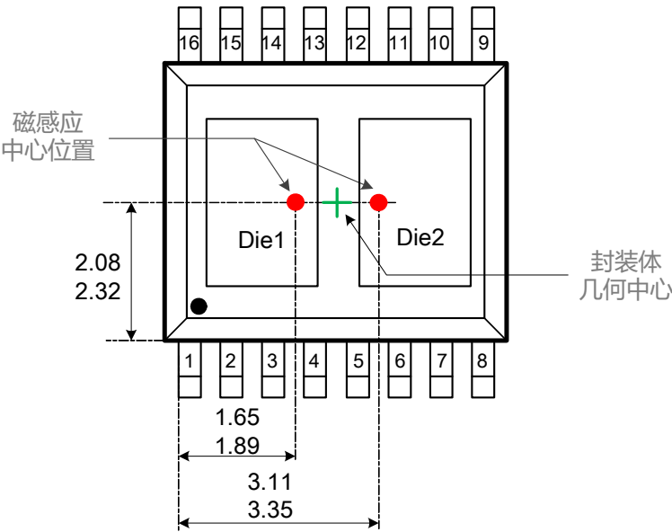
图-2: TSSOP-16 封装
