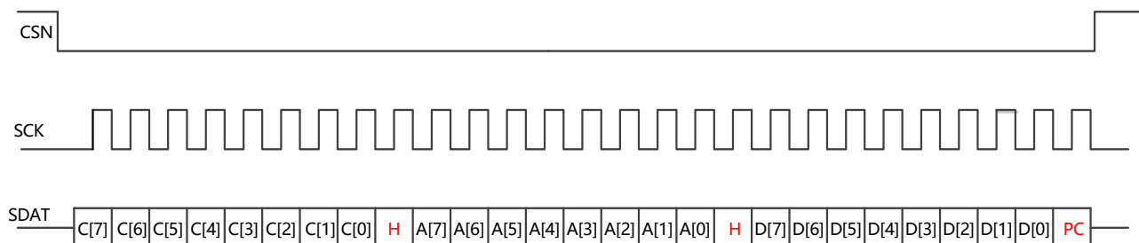
图-12: 3线SPI接口
