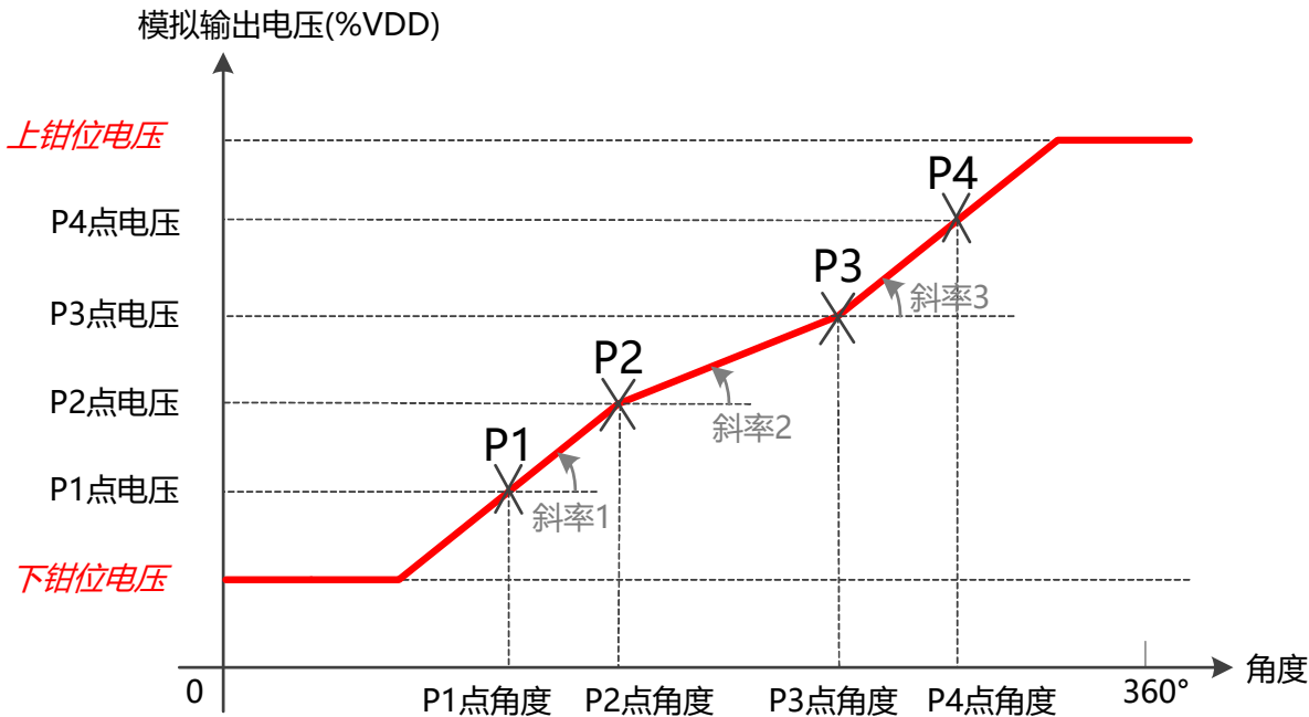
图-11: 模拟输出4点和上、下钳位电压编程
