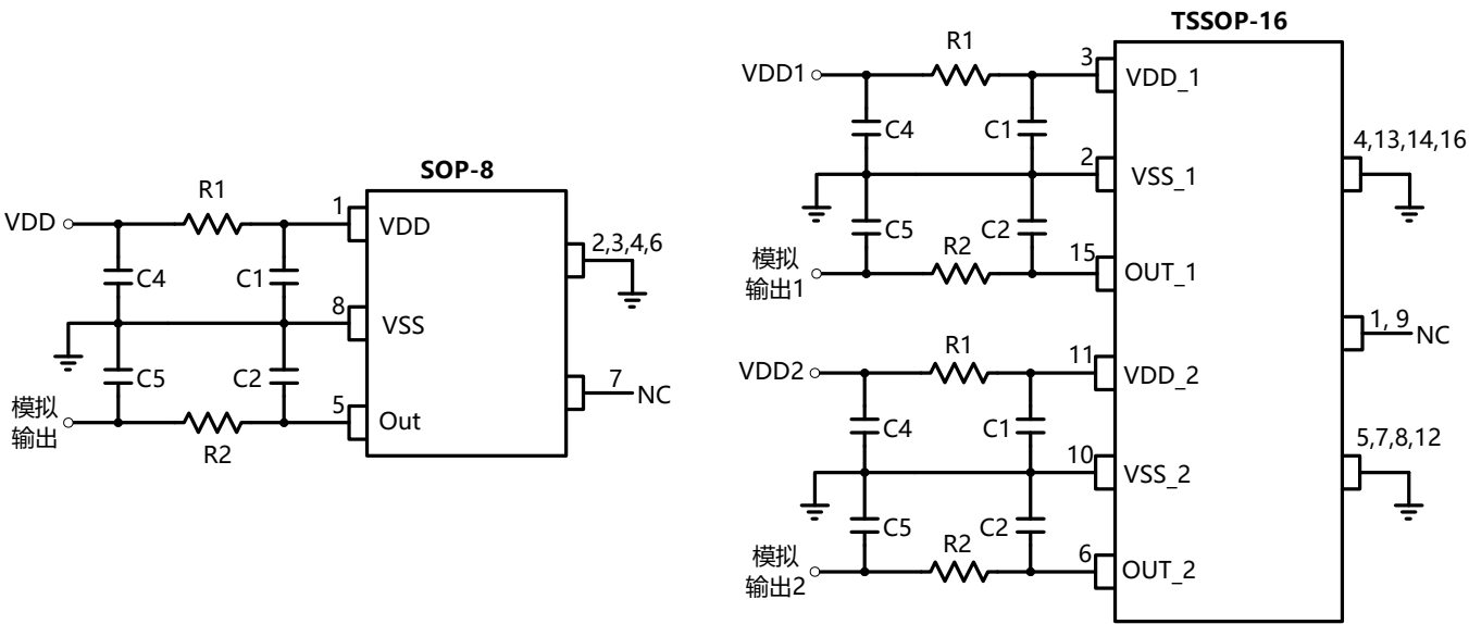
图-14: 模拟输出参考电路
