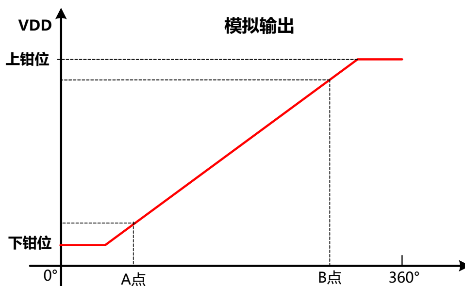
图-6: 模拟输出
