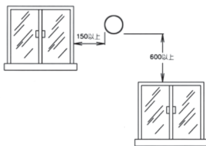
排气管出口距进风口距离
