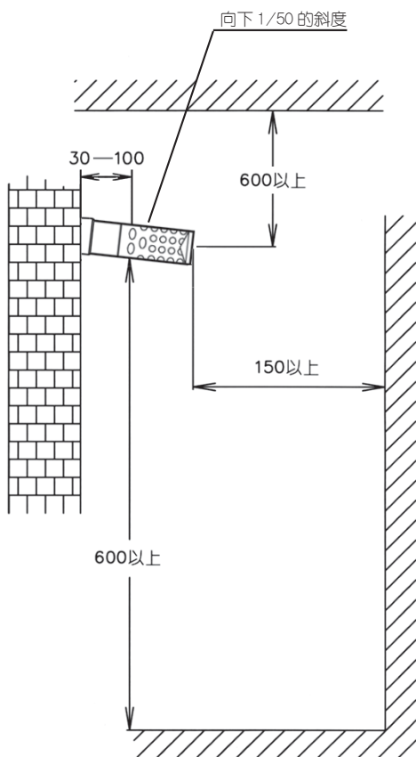
排气管出口侧面
