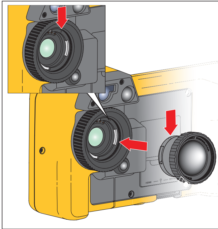
图 2. 可选镜头安装
