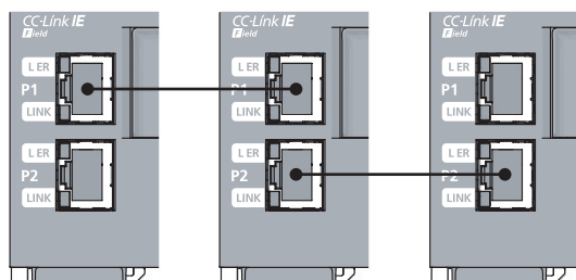
PORT1之间、PORT2 之间的连接
