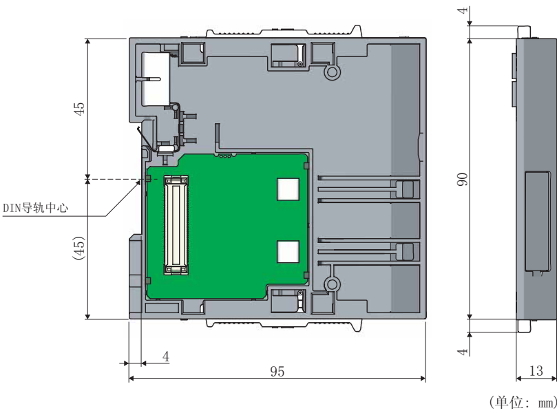
(2) END 盖板 (L6EC)
